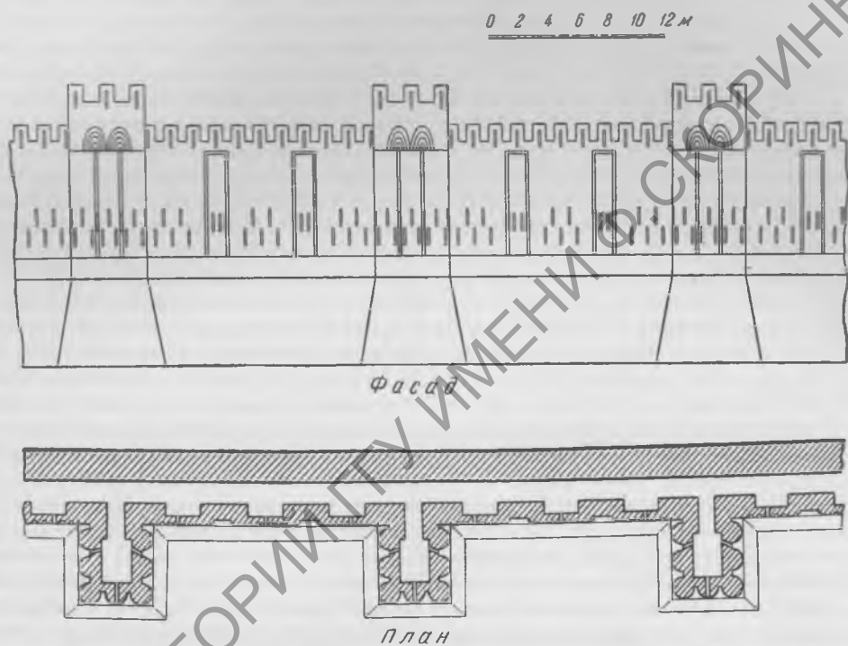
Рис. 6. Парфянская крепость «Чильбурдж» (чертежи реконструкции стен)
