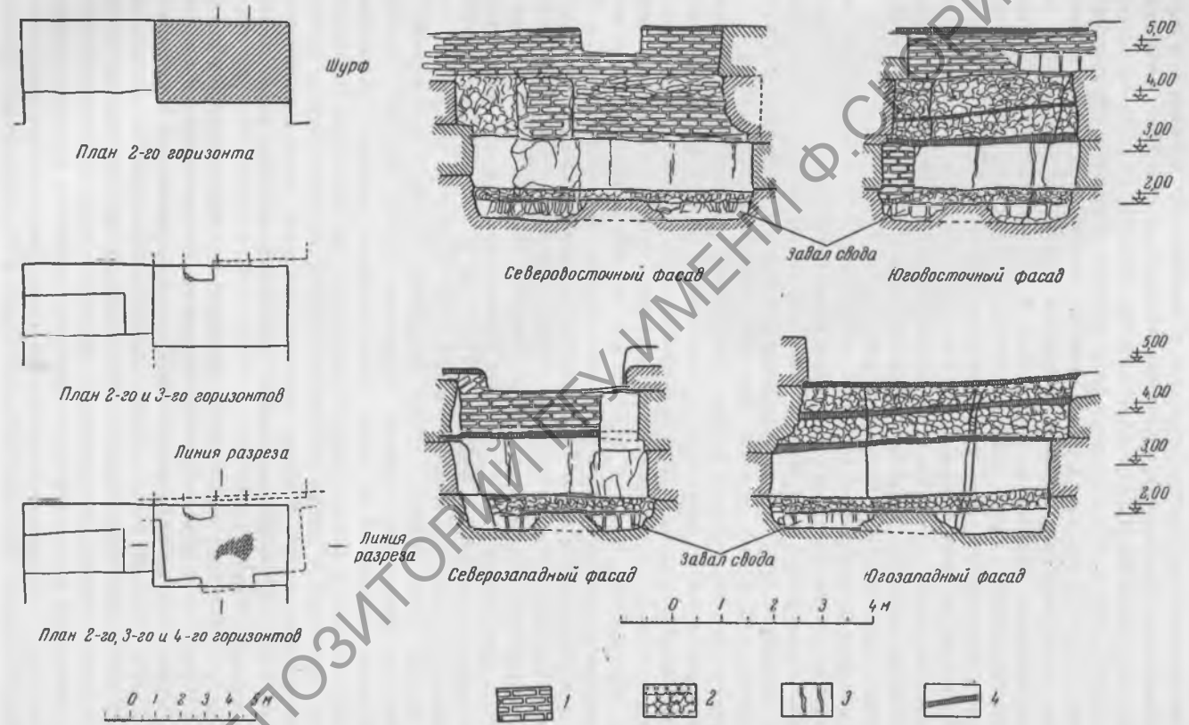
Рис. 4. Купя-Уз. Стратиграфический разрез на одном из участков городища. Условные обозначения: 1 — сыровые кирпичи; 2 — завал; 3 — пахса; 4 — почвы
