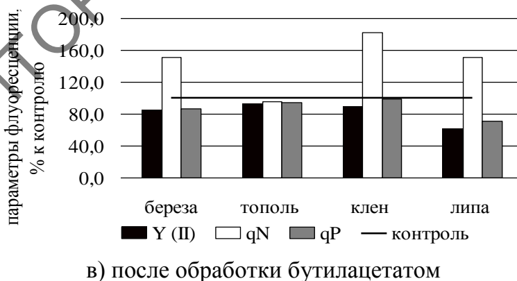
Рисунок 2 – Изменение значений Y(II) , qP и qN в листьях саженцев древесных растений (представлены усредненные значения изменений в пределах всех доз каждого соединения)
