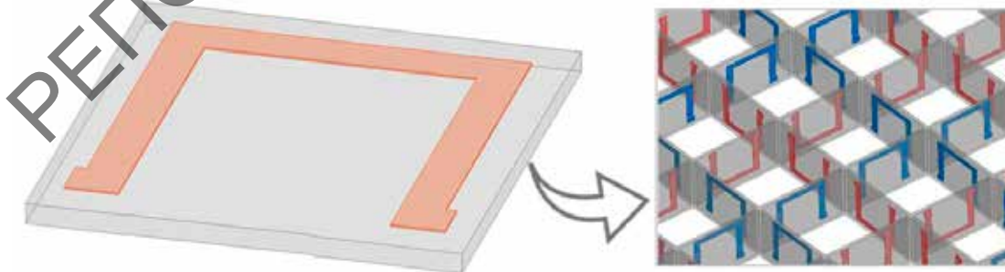
Рис. 2. Схема конструирования трехмерного образца метаматериала из плоских омега-резонаторов прямоугольной формы на подложке
