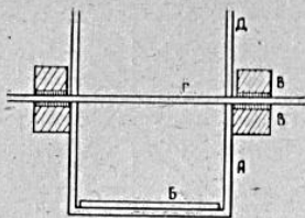
Рис. 3. Схема дополнительного приспособления к приставке: А — корпус приспособления, Б — зеркало, В — кольцевые магниты, Г — стекло, Д — корпус приставки
