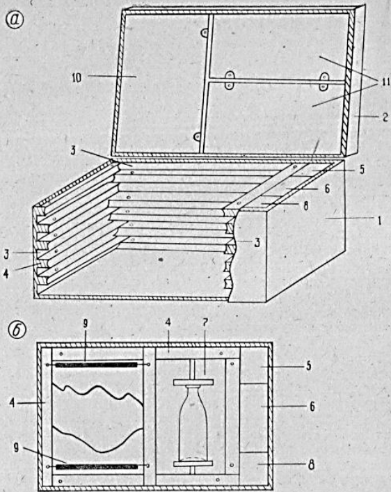
Рис. 1. Контейнер «КУВеД»: а) разрез контейнера, б) вид сверху
