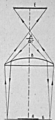
Рис. 2. Оптическая схема приставки применительно к освещению следа в отраженном свете: А — след, Б — следовоспринимающая поверхность, В — объектив, Г — источник света, Д — непрозрачный экран, Е — фотопленка
