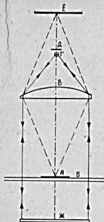
Рис. 1. Оптическая схема приставки применительно к освещению следа методом темного поля: А — след, Б — стекло, В — объектив, Г — источник света, Д — непрозрачный экран, Е — фотопленка, Ж — зеркало
