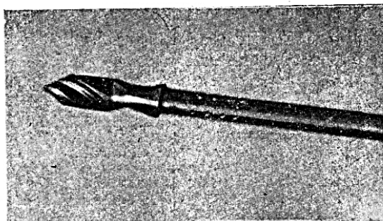
Рис. 1. Наконечник шупа в форме сверла
