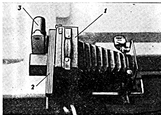
Рис. 3. Установка для репродукционной съемки 1 — «Фотокор», 2 — фотоприставка, 3 — «ФЭД»
