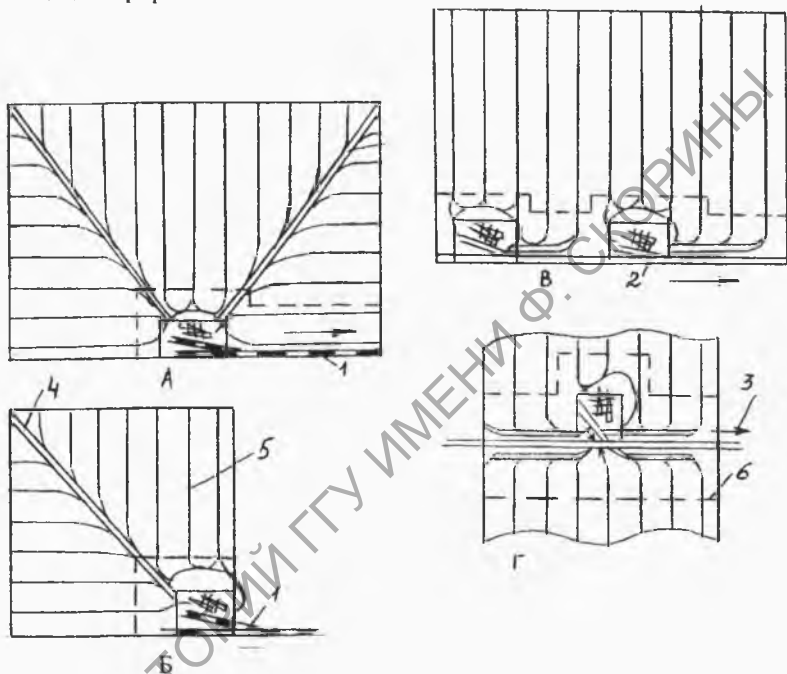
Рисунок 1 – Транспортная сеть на лесосеках компактной формы площадью более 5 га (А), менее 5 га (Б) и на узких лесосеках (В, Г): 1 – вывозка железной дорогой; 2 – автовывозка; 3 – направление вывозки; 4 – волоки магистральные; 5 – волоки пасечные; 6 – зона безопасности (по Тихонову А. С. (16)).
