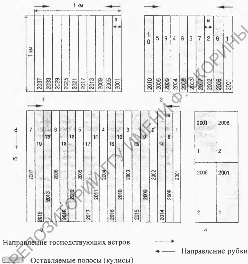
Рисунок 2 – Примыкание лесосек: 1 – непосредственное; 2 – чересполосное; 3 – кулисное; 4 – шахматное (а – ширина лесосеки; 1.....19 – № лесосек, 2001 –2037 – год рубки)
