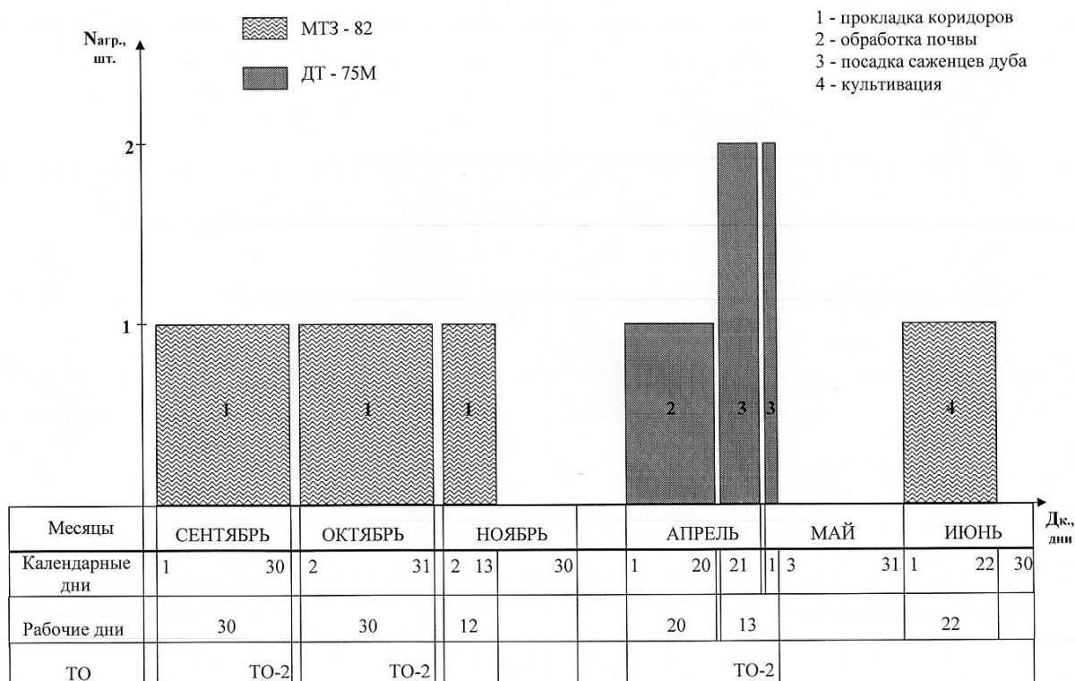
Рисунок 1 – График машиноиспользования
