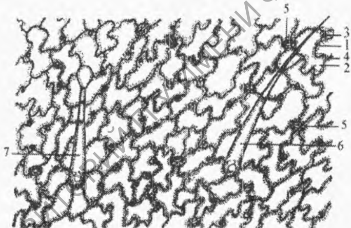
Рисунок 2.4 – Эпидермис листа герани ( Pelargonium zonale ): 1 – оболочка клетки, 2 – цитоплазма, 3 – ядро, 4 – хлоропласты, 5 – устьица, 6 – простой волосок, 7 – железистый волосок (из Н. С. Киселева, Н. В. Шелухин, 1969)
