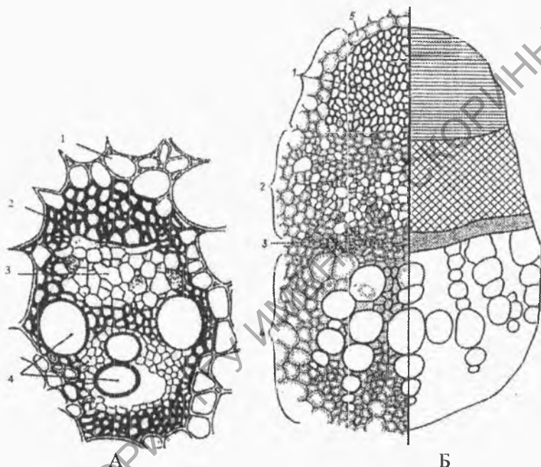
Рисунок 4.3 - Коллатеральные пучки: А - Коллатеральный закрытый сосудисто-волокнистый проводящий пучок стебля кукурузы ( Zea mays ) в поперечном разрезе: 1 – основная паренхима, 2 – склеренхима, 3 – протофлоэма, 4 – метафлоэма, 5 – древесная паренхима, 6 – пористые сосуды, 7 – спиральный сосуд, 8 – кольчатый сосуд, 9 – воздушная полость (из Н. С. Киселева, Н. В. Шелухин, 1969); Б - Коллатеральный открытый сосудисто-волокнистый проводящий пучок стебля подсолнечника ( Helianthus annuus ) в поперечном разрезе: 1 – основная паренхима, 2 – склеренхима, 3 – флоэма, 4 – камбий, 5 – вторичная ксилема, 6 – первичная ксилема, 7 – перимедулярные волокна (из Н. С. Киселева, Н. В. Шелухин, 1969)
