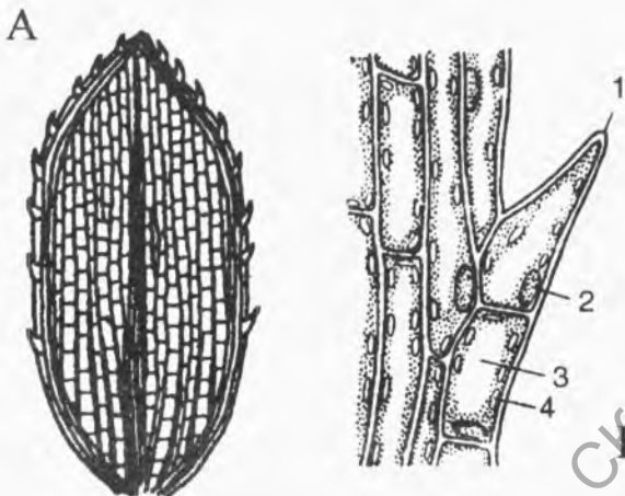
Рисунок 1.1 – Лист элодеи канадской ( Elodea canadensis ):
