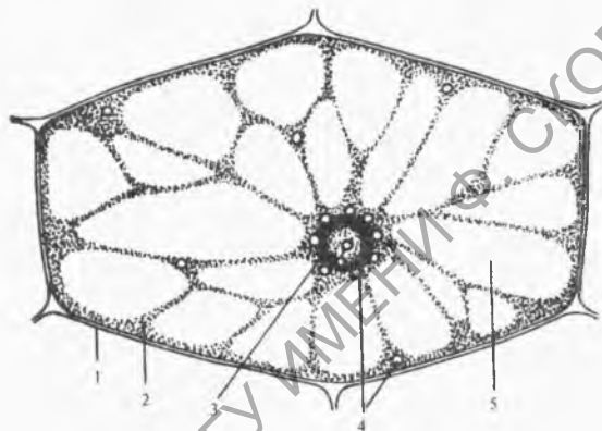
Рисунок 1.3 – Лейкопласты в клетках кожицы листа традесканции ( Tradescantia virginiana : 1 – оболочка, 2 – цитоплазма, 3 – ядро, 4 – лейкопласты, 5 – вакуоля (из Г. А. Бавтуго, 2001)
