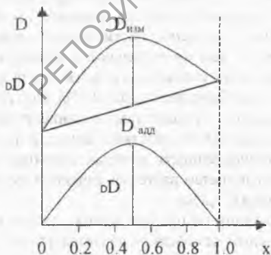
рис. 1 График зависимости оптической плотности от состава комплекса.
