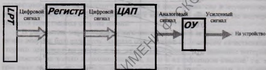
Рис. 1. Функциональная схема генератора аналоговых сигналов.
