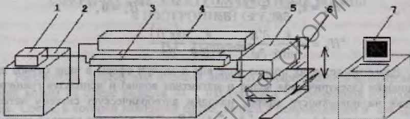
Рисунок. Схема макета установки для лазерной обработки неметаллических материалов.
