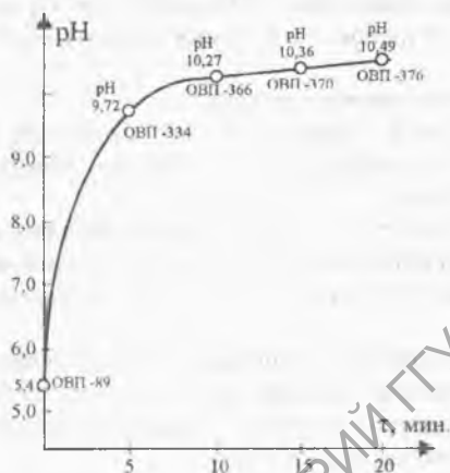
Рисунок 1 Динамика изменения рН и значения ОВП католита в зависимости от времени ЭХА.
