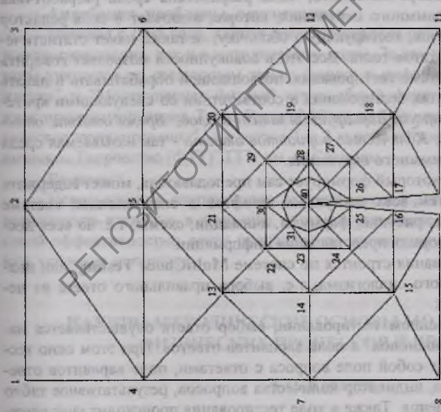
Рис 1. Начальное разбиение образца на КЭ (нулевое приближение). Узел номер 40 – устье трещины.
