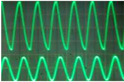
Рисунок 7 – Осциллограммы сигналов на излучающем элементе и приемнике акустических волн
