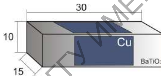
Рисунок 2 – Линейные размеры изготовленного акустического волновода
