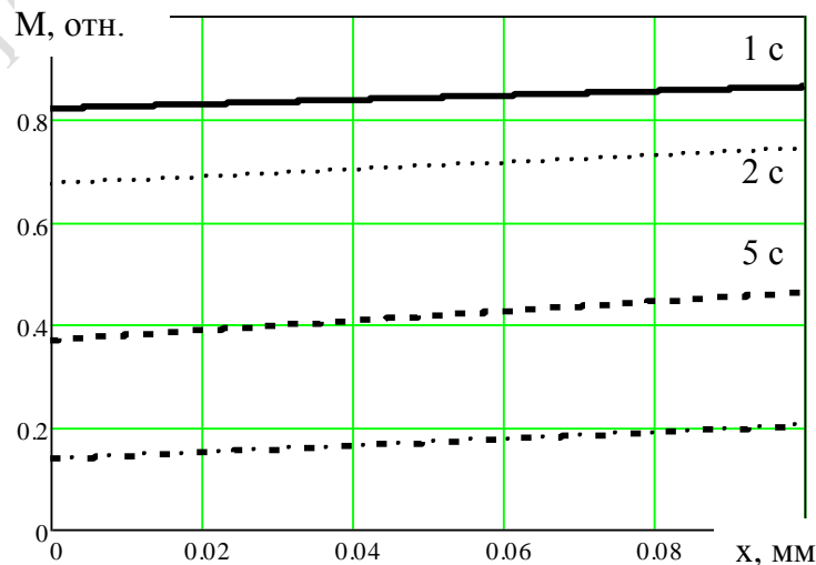
Рисунок 3 – Зависимость нормализованной концентрации светочувствительного компонента от толщины слоя фоторезиста, рассчитанная для различного времени экспозиции
