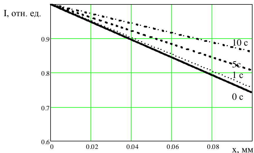
Рисунок 4 – Зависимость относительной интенсивности излучения от толщины слоя фоторезиста, рассчитанная для различных времен экспозиции
