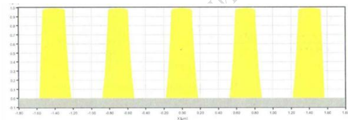
Рисунок 2 – Изображение профиля фоторезистивной маски структуры элемент/зазор 0,35 мкм, полученное в результате компьютерного моделирования
