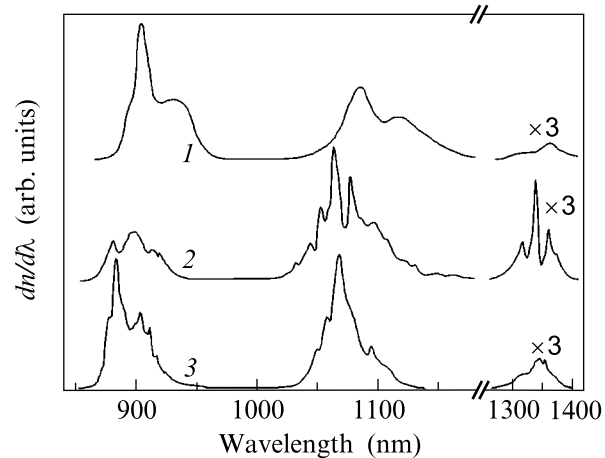
Рис.2. Нормированные и корректированные спектры ИК-люминесценции Nd- (1) и Ce-Nd-содержащих стекол до (2) и после (3) отжига в водороде; N_{Nd} , 10^{19} ионов/см 3 : 2 (1), 15 (2, 3), N_{Ce} = 3 \cdot 10^{20} ионов/см 3 (2, 3), \lambda_{exc} , нм: 300–750 (1), 370 (2, 3)
