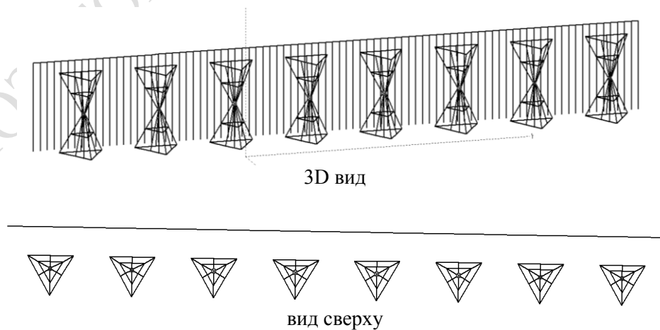
Рисунок 2 – Антенная решетка перед вертикальным рефлектором
