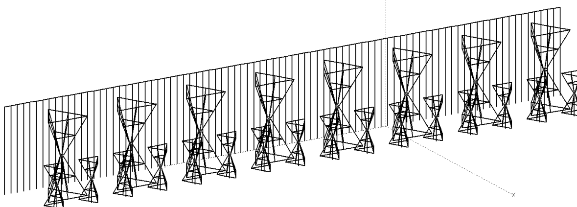
Рисунок 8 – Двухлитерный совмещенный вариант антенной решетки
