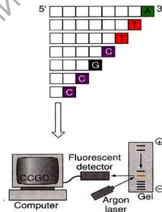
Рисунок 108. Автоматическое секвенирование.
