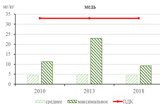
Рисунок 3 – Содержание контролируемых химических ингредиентов в почвах г. Солигорск. Составлен по данным [5]
