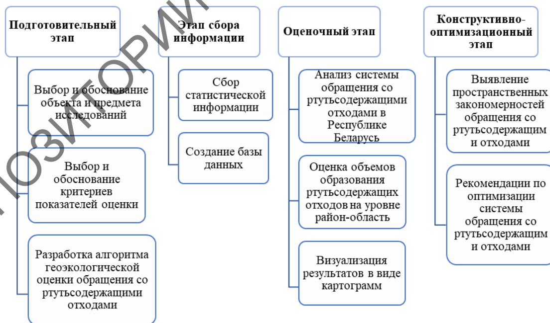
Рисунок 1 – Алгоритм геоэкологической оценки обращения со ртуťсодержащими отходами в Республике Беларусь
