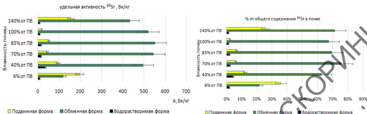
Рисунок 2 – Содержание ^{90}\text{Sr} в водорастворимой, обменной и подвижной формах в образцах аллювиальной (пойменной) дерново-глебоватой почвы в зависимости от влажности почвенной среды
