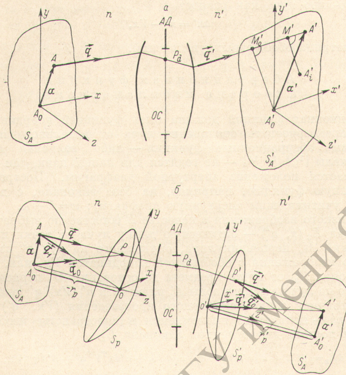
Рис. 1. Обобщенные координаты на предмете и изображении.
