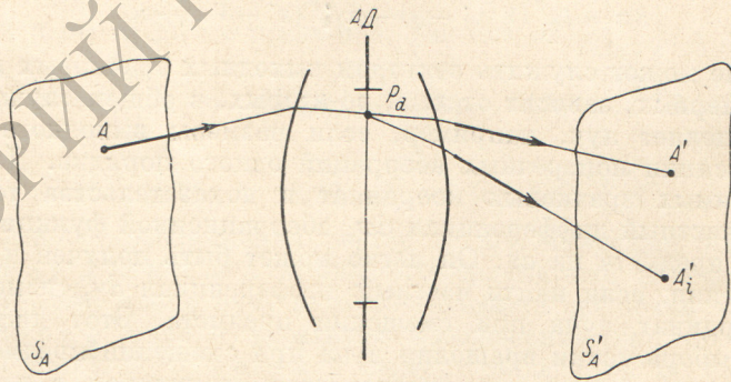
Рис. 2. К геометрической интерпретации aberrационной функции и зрачковых координат.
