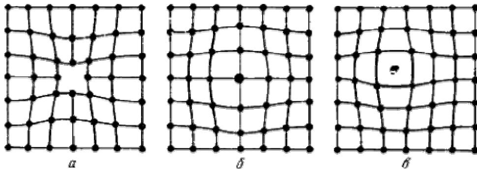
Рис.2.1. Точечные дефекты
