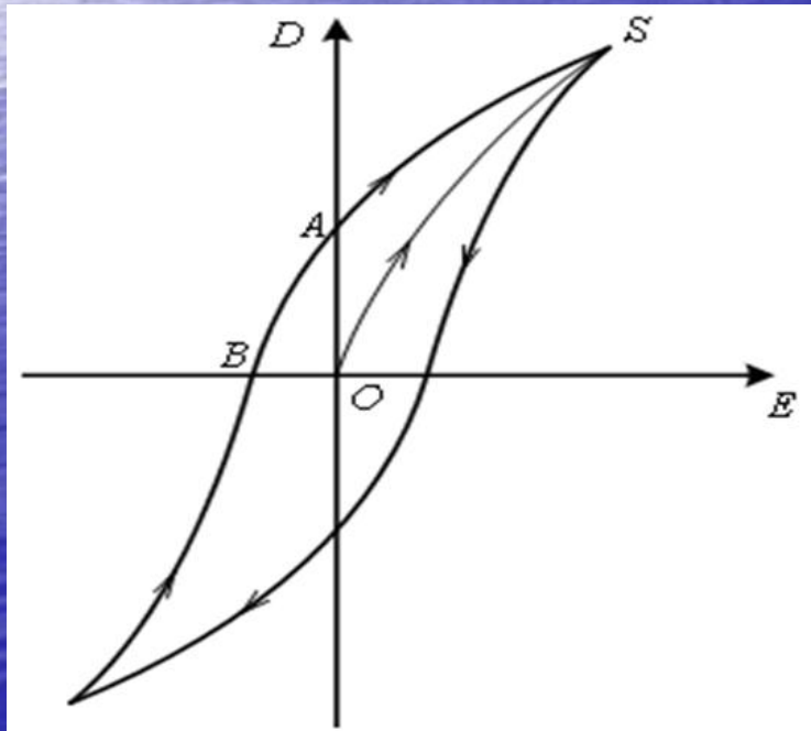
Рис.4-Зависимость электрической индукции от напряжённости для сегнетоэлектрика(петля гистерезиса)
