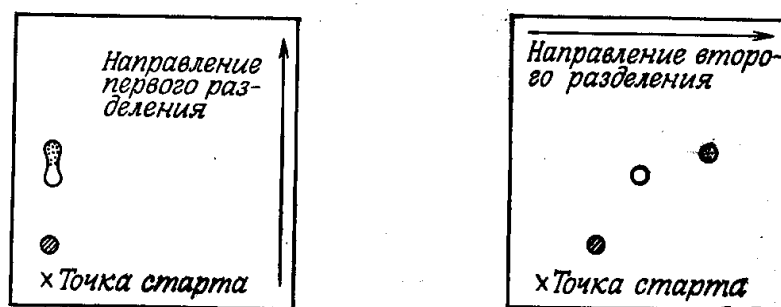
Рис. 3. Двухмерная хроматограмма
