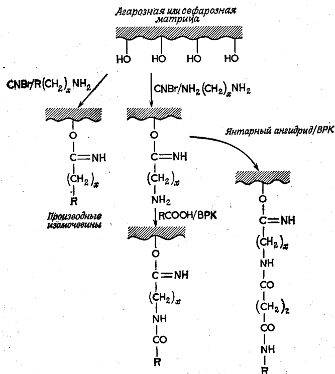
Рис. 8. Возможные пути сшивания лиганда с агарозой или сефарозой. Буквой R обозначен лиганд, с которым связывается макромолекула, символом ВРК обозначен водорастворимый карбодиимид. Для простоты приведена реакция только с одной из гидроксильных групп.
