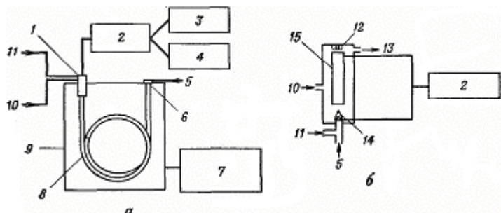
Рис.5. Схема устройства прибора для газожидкостной хроматографии (а) и пламенно-ионизационного детектора (б)
