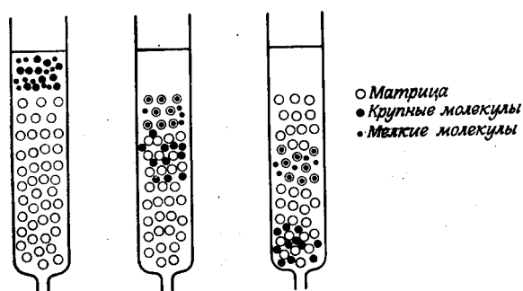
Рис. 7. Разделение веществ методом проникающей хроматографии
