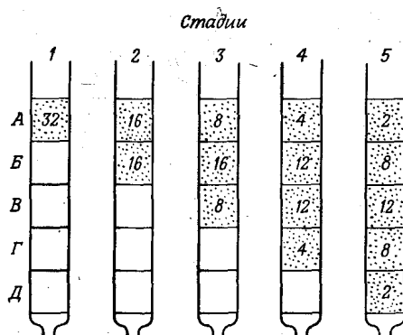
Рис. 2. Схема разделения веществ (теория теоретических тарелок)
