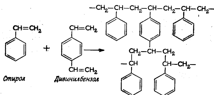
Рис. 6. Сополимеризация стирола и дивинилбензола
