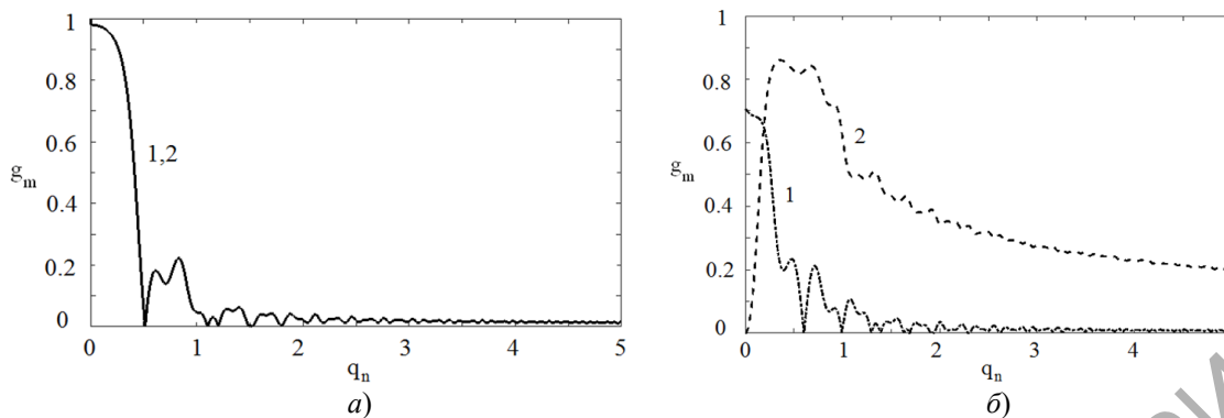
Рисунок 2.1 – Зависимость интеграла перекрытия g_{\pm,\pm} \equiv g_m от параметра q_n = q/q_0 для дифракции бesselевого пучка нулевого порядка (а) и первого порядка (б); анизотропная дифракция (кривая 1, 2-правополяризованная в левополяризованную (и наоборот) максимум g_m = 0,98 для m = 0 ); (б) дифракция правополяризованной волны в левополяризованную (кривая 1) максимум g_m = 0,72 для m = 1 ; дифракция левополяризованной в правополяризованную (кривая 2) максимум g_m = 0,87 для m = 1 (кристалл TeO_2 ; медленная сдвиговая УЗ волна распространяется под малым углом \delta к оси X||[110] ; \gamma_{\pm} = 0,5^0 , \beta = 83 град/мм, R_B = 1 мм, \lambda_0 = 0,63 мкм)
