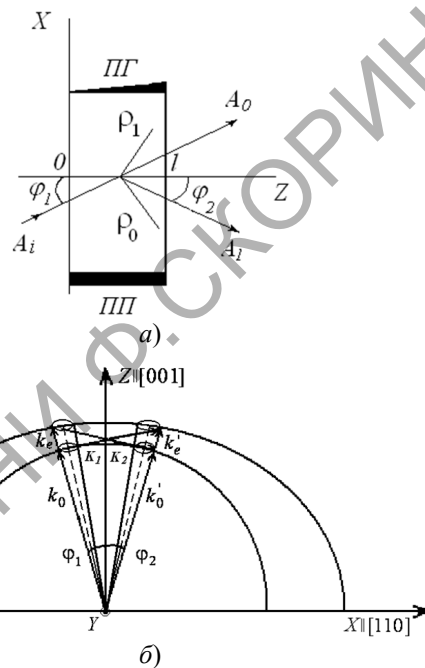
Рисунок 1.1 – а) Схема АО взаимодействия БСП и УЗ волны (ПП – пьезопреобразователь, ПГ – поглотитель ультразвука, \varphi_1 и \varphi_2 – угол падения и дифракции соответственно); б) геометрия расположения преломленной и дифрагированной плосковолновых компонент БСП в плоскости дифракции на медленной сдвиговой УЗ волне в кристалле TeO_2 ( \vec{K}_{1,2} – волновые векторы ультразвука, \vec{k}_{o,e} , \vec{k}'_{o,e} – волновые векторы преломленной и дифрагированной волн)
