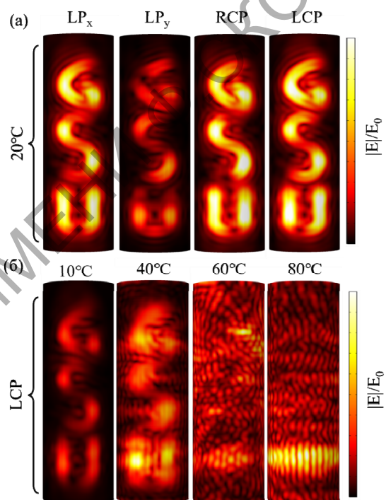
Рисунок 3.2 – Результаты моделирования напряженности электрического поля в ближней зоне при различной поляризации падающей волны (a) и распределение поля при различных температурах (б)
