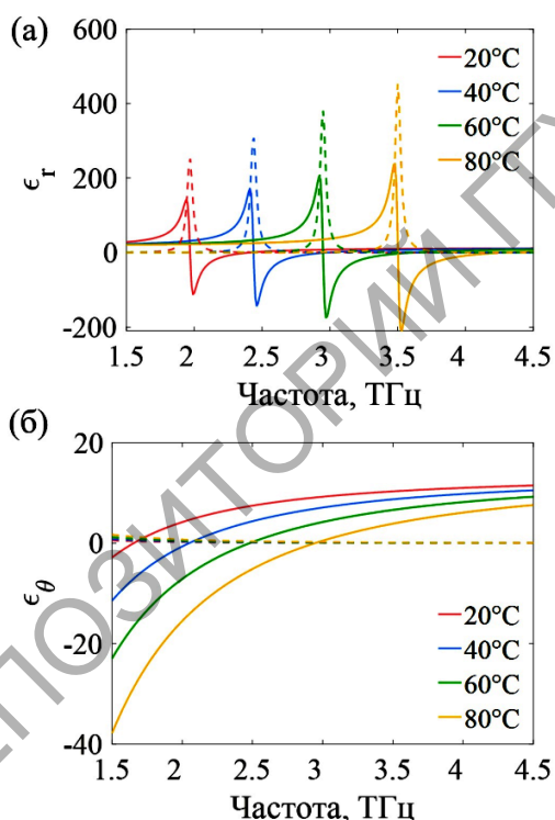
Рисунок 3.1 – Радиальная \epsilon_r (a) и азимутальная \epsilon_\theta (б) диэлектрическая проницаемость гиперлинзы при разных температурах
