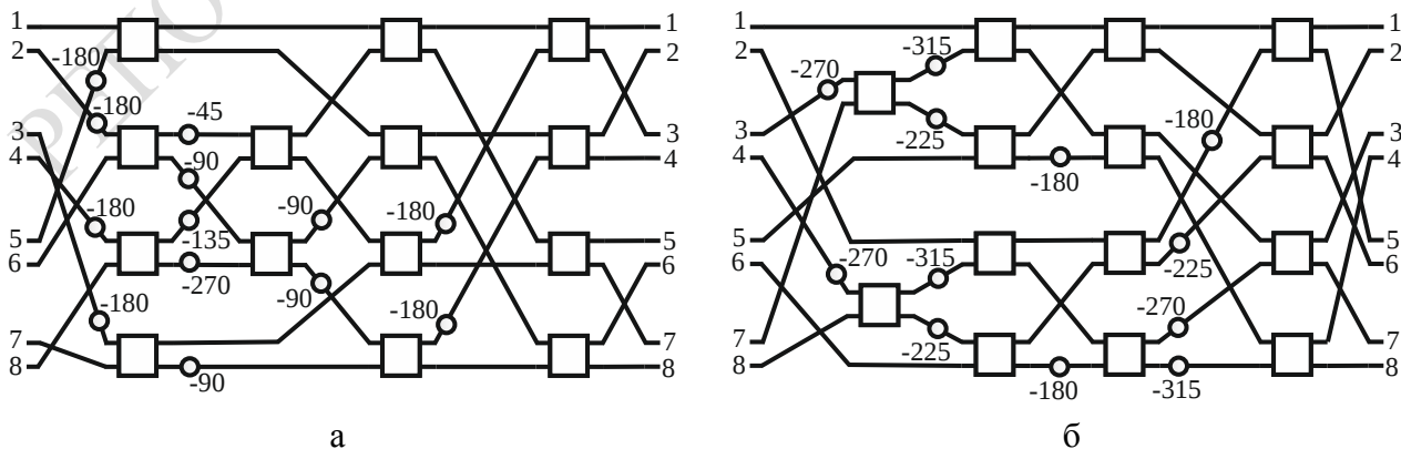
Рисунок 8. – Синтезированные диаграммообразующие схемы 8 \times 8 выходов
