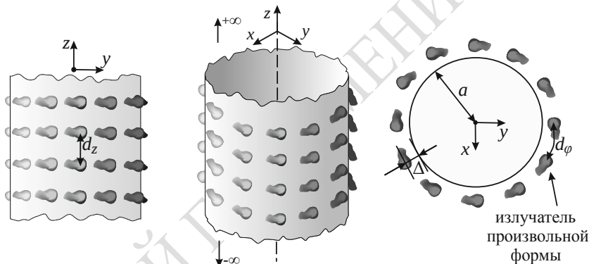
Рисунок 1. – Бесконечная антенная решетка излучателей над идеально проводящим круговым цилиндром
