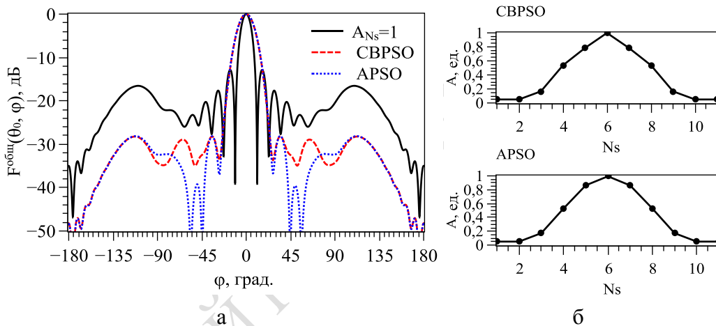
Рисунок 4. – Характеристики направленности антенной решетки при двух синтезированных амплитудных распределениях
