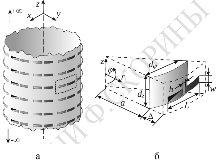
а – антенная решетка; б – модель излучателя
