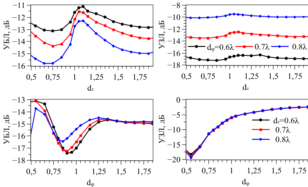
Рисунок 6. – Зависимости выходных характеристик антенной решетки от периодов
