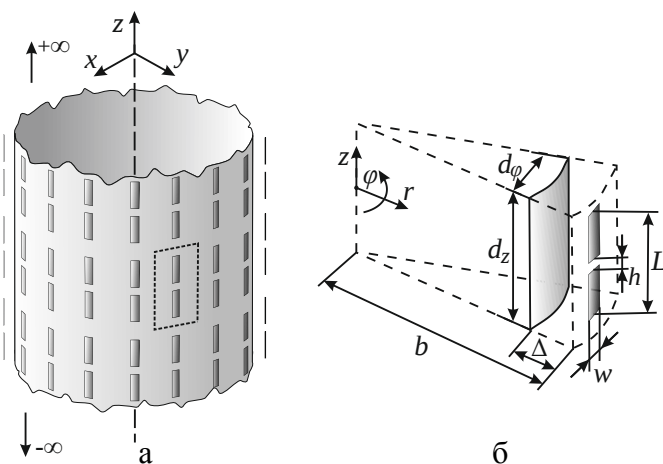
а – антенная решетка; б – модель излучателя
