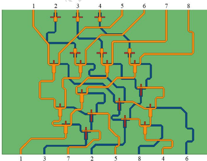
Рисунок 10. – Топология диаграммообразующей схемы в печатном исполнении
