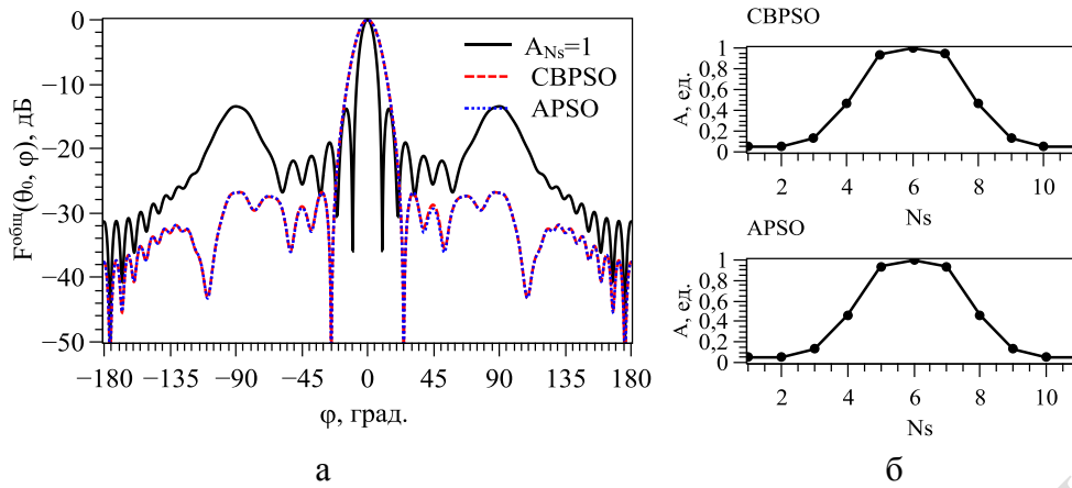
а – диаграммы направленности; б – амплитудные распределения
