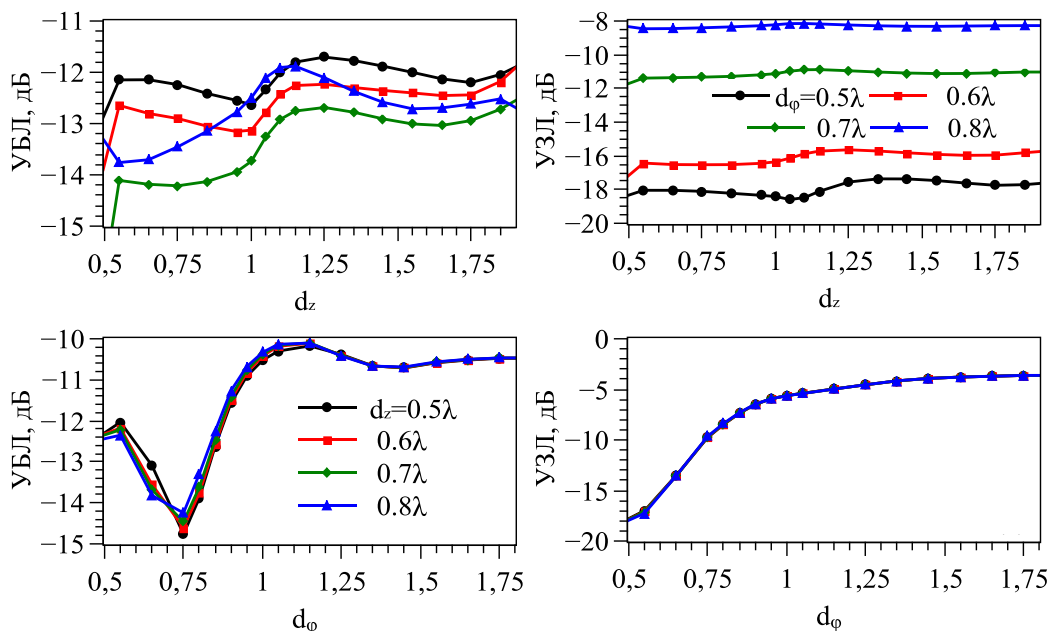
Рисунок 3. – Зависимости уровня боковых и задних лепестков фазированной антенной решетки от периодов антенной решетки ( N=32 , \alpha=120^\circ )
