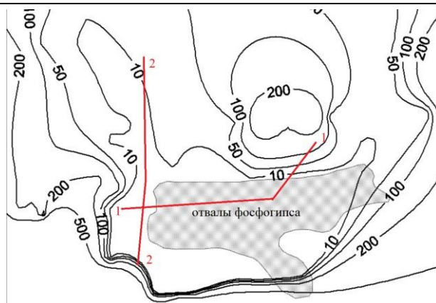
Рис. 2. Изолинии кажущегося электрического сопротивления (Ом м) на эффективной глубине, соответствующей разному AB=3 м. Таким образом, химическое загрязнение верхней части геологической среды на территории отвалов фосфогипса и в зоне их влияния фиксируется аномалиями низкого кажущегося электрического сопротивления, измеряемого на разносах питающих электродов 3-10 м.
