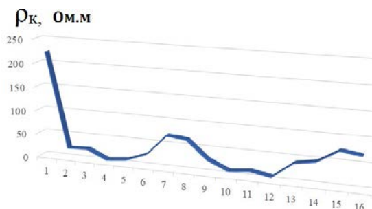
Рис. 4. Изменения кажущегося электрического сопротивления по профилю 2 (AB=10 м)
