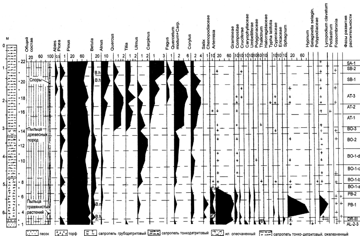
Рисунок 2 – Пыльцевая диаграмма отложений голоценового межледниковья в оз. Ореховское (скв., Беларусь). Анализ Я. К. Еловичевой
