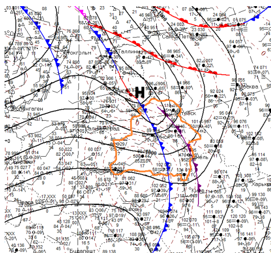
Рисунок 1 – Приземная синоптическая ситуация за 04.11.2013 г. 03 UTC при возникновении очень сильного ветра в Верхнедвинске
