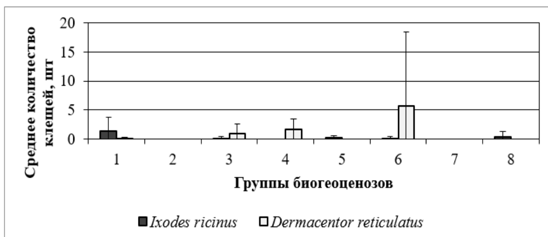
Рисунок 3 – Встречаемость клещей в различных биогеоценозах
