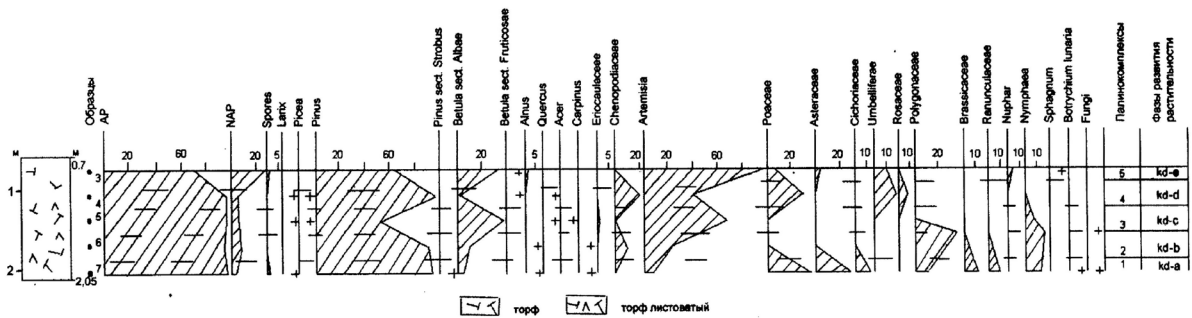
Рисунок 6 – Пыльцевая диаграмма отложений шкловского/кайдаковского Межледникового у г. Канев (скв. 2-а, Украина). Анализ Я. К. Еловичевой
