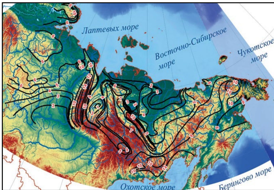
Рисунок 1 – Карта модуля годового стока по данным до 2017 г. [4]
