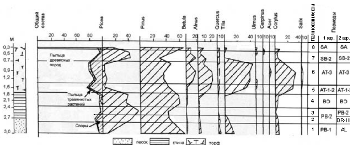
Рисунок 1 – Пыльцевая диаграмма отложений голоценового межледниковья в оз. Долгое (скв., Украина). Анализ Е. И. Шириной
