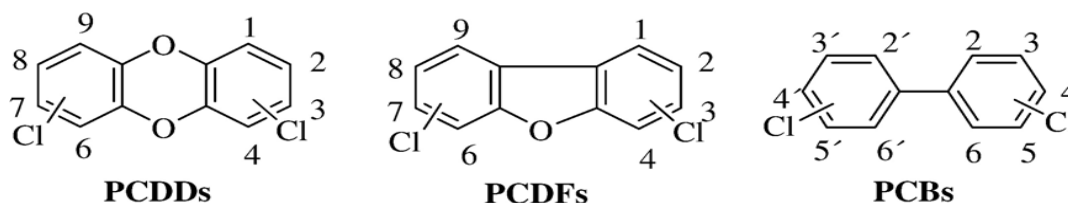
Рисунок 1 – Структурные формулы хлорсодержащих диоксинов, фуранов и бифенилов. Нумерация относится к атому углерода, доступному для замещения хлором
