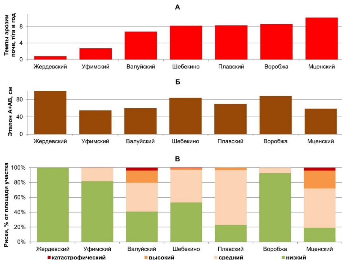
Рисунок 1 – Осредненные по участкам темпы эрозии почв (А); эталонные мощности несмытых почв (Б); риски деградации земель от водной эрозии почв, выраженные в виде долевого участия суммарных площадей полей с указанными рисками относительно общей площади участков (В)
