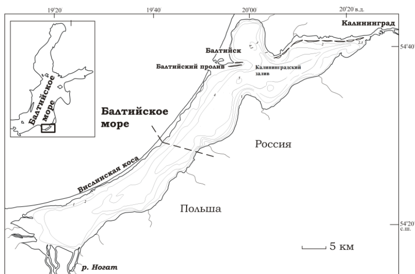
Рисунок 1 – Расположение Калининградского залива
