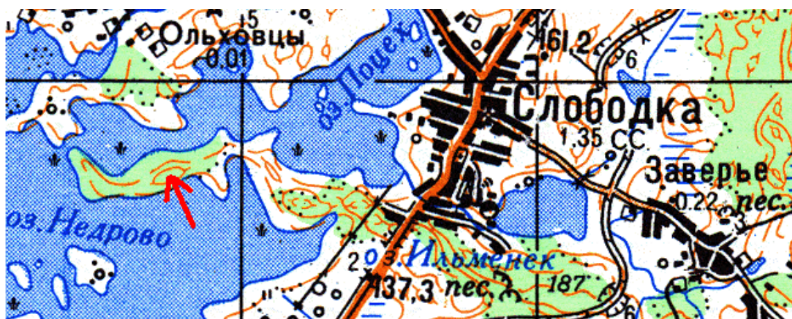
Рисунок 2 – Схема расположения высшей точки Слободковской гряды
