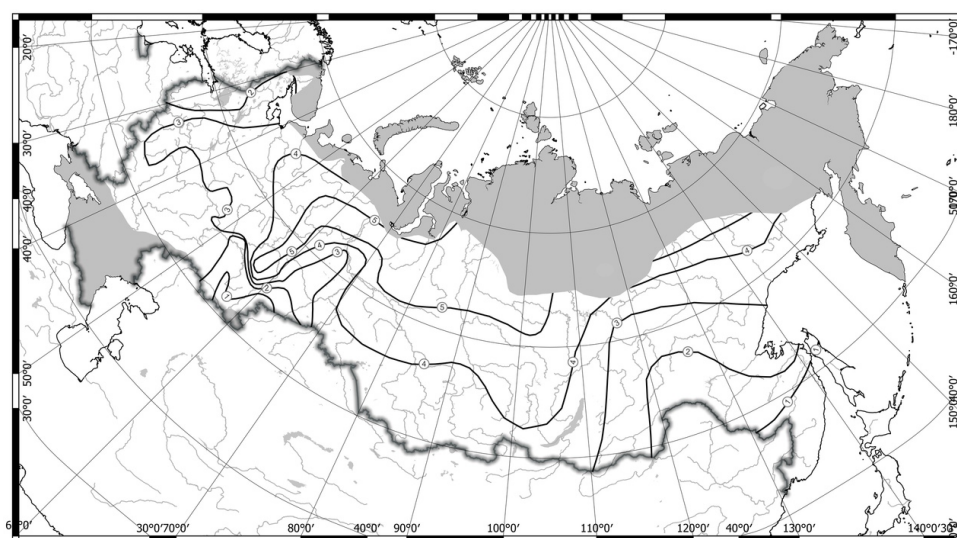
Рисунок 1 – Изофены осеннего состояния березы пушистой и бородавчатой на территории РФ 15 сентября 2023 года
