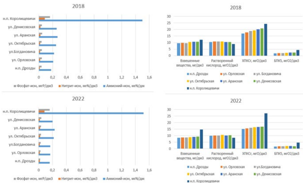
Рисунок 1 – Показатели загрязняющих веществ в р. Свислочь по результатам наблюдений НСМОС
