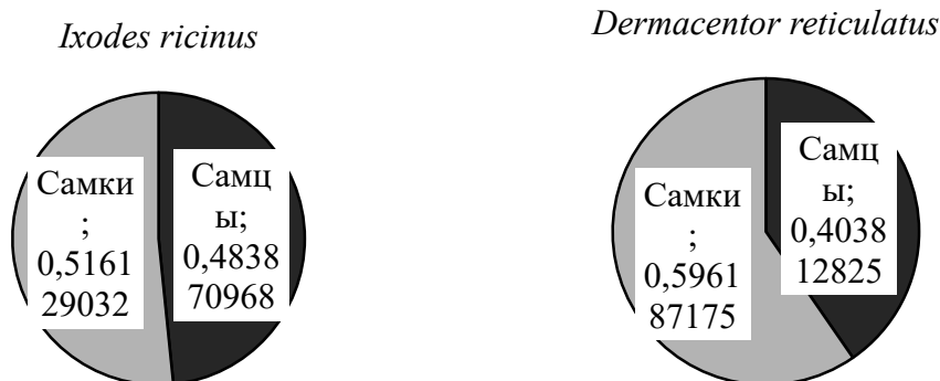
Рисунок 3 – Половая структура популяций клещей
