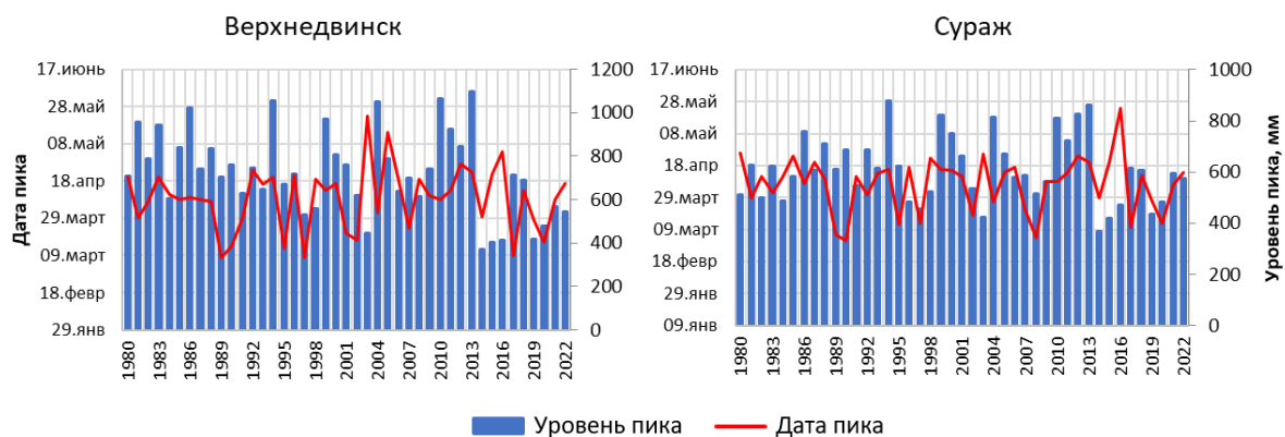
Рисунок 3 – Даты и уровни пика половодья в створе гидропоста Верхнедвинск и Сураж за период 1980–2022 гг. (построено по данным [1])
