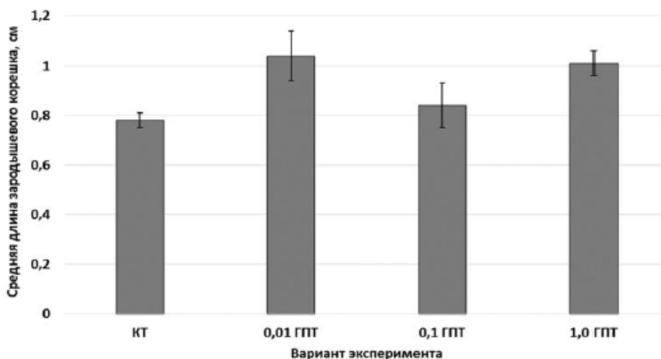
Рисунок 2 – Изменение средней длины зародышевых корешков тест-культуры в условиях смоделированного низкотемпературного стресса
