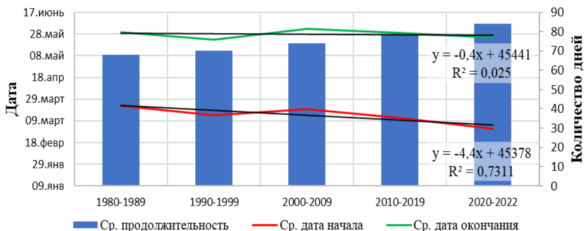
Рисунок 2 – Усреднённые даты начала и окончания половодья и его продолжительность по десятилетним срезам (построено по данным [1])
