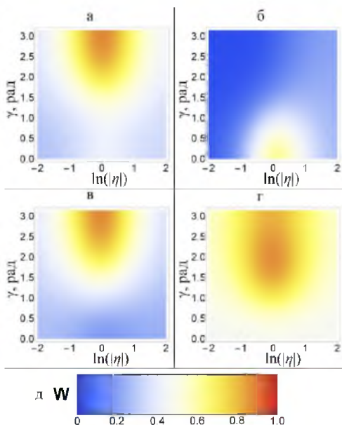
Рис. 1. Зависимость полной мощности ГВГ-СЧ от угла раскрытия и модуля отношения комплексных амплитуд при \arg \eta = -1,5 рад. Легенда представлена на рисунке 1 д. На фрагментах а–г представлены графики для следующих типов анизотропии: (а) – \chi_1^{(2)} , (б) – \chi_2^{(2)} , (в) – \chi_3^{(2)} , (г) – \chi_4^{(2)}
