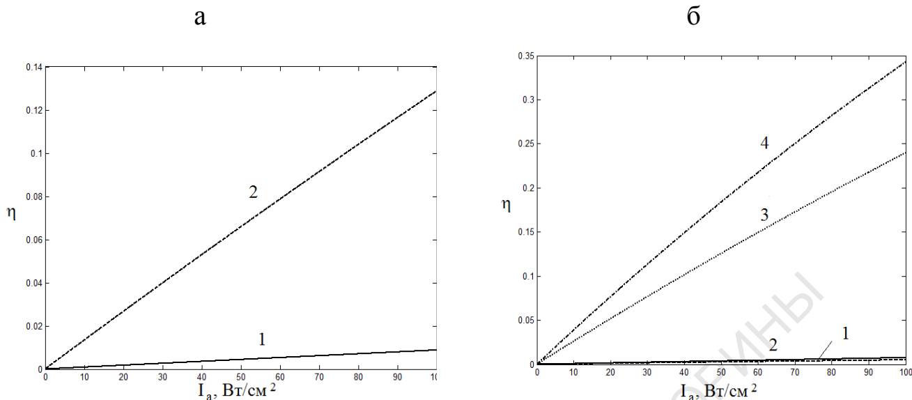
Рисунок 2 – Зависимость эффективности дифракции \eta от интенсивности ультразвука для падающего БСП нулевого порядка (а) и первого порядка (б); а) изотропная дифракция (1), анизотропная дифракция (2); б) дифракция правополяризованной волны в левополяризованную (1), левополяризованной в левополяризованную (2), правополяризованной в правополяризованную (3), левополяризованной в правополяризованную (4) (кристалл \text{Bi}_{12}\text{GeO}_{20} , продольная УЗ волна, \vec{K} \parallel [100] , m=0 (а), m=1 (б), \gamma_0=0,5^\circ , \rho=22 град/мм, R_H=1 мм, l=5 см; интегралы перекрытия: g_{+,+} = g_{-,-} = 0,53 , g_{-,+} = g_{+,-} = 0,98 (а); интегралы перекрытия: g_{-,+} = g_{-,-} = 0,93 , g_{+,-} = g_{+,+} = 0,76 (б))
