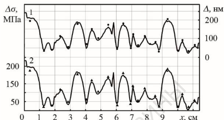
Рисунок 2 – Распределение механических напряжений \sigma и оптической разности хода \Delta в плоскости стекла; ● и ▲ – данные ПКС 250
