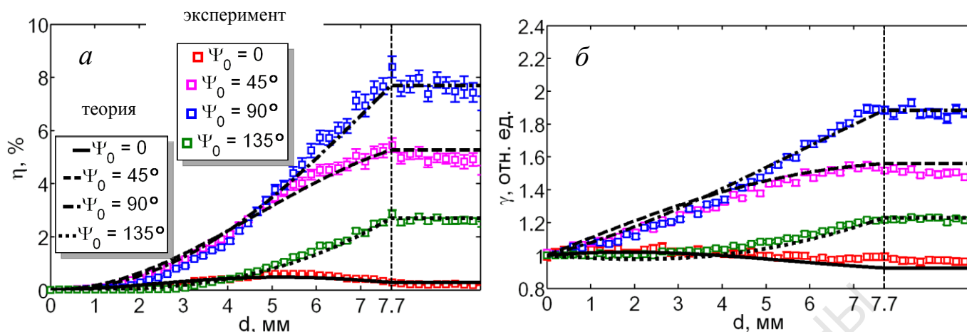
Рисунок 1 – Зависимости дифракционной эффективности \eta голограмм (а) и коэффициента усиления \gamma предметной световой волны (б) от толщины d кристалла ВТО среза (\bar{1}\bar{1}0)
