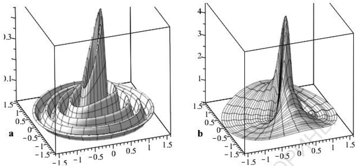
Рисунок 1 – 3D графики интенсивности aV -мод при \nu = 1,5 ; x_0 = 0 ; \alpha = 10 ; слева а) y_0 = 0,05i , справа б) y_0 = 0,2i
