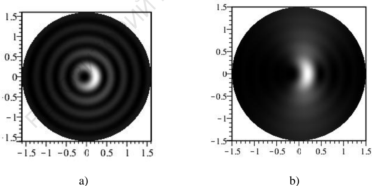
Рисунок 2 – 2D графики интенсивности aV -мод при \nu = 1,5 ; x_0 = 0 ; \alpha = 10 ; слева а) y_0 = 0,05i , справа б) y_0 = 0,2i
