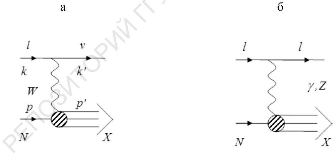
Рисунок 1 – Процессы lN -ГНР с заряженным (а) и нейтральным (б) токами в борновском приближении
