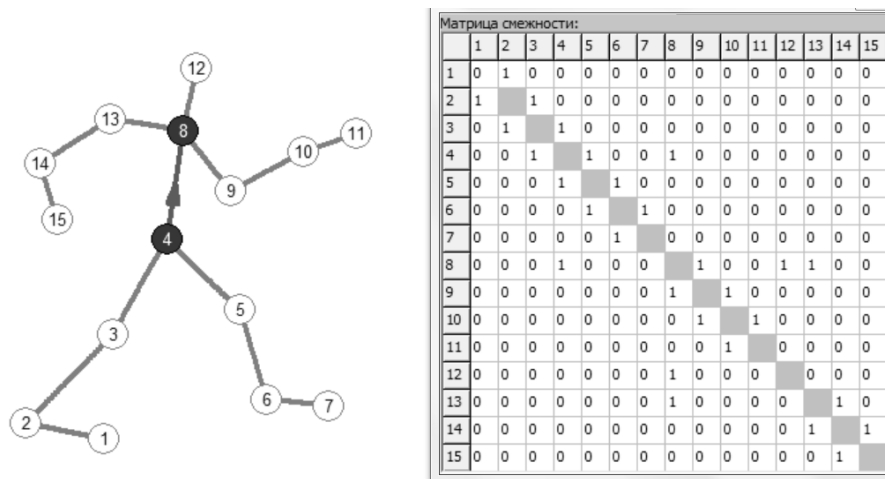
Рисунок 2 – Ориентированный граф и матрица смежности 15-ти звенной модели опорно-двигательного аппарата тела человека
