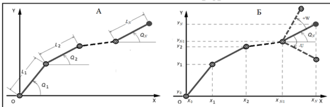
Рисунок 1 – Обозначения в кинематической схеме многозвенной модели биомеханической системы
