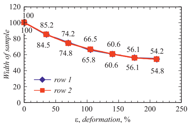
Рис. 4. Изменение ширины образцов в процессе деформации.
