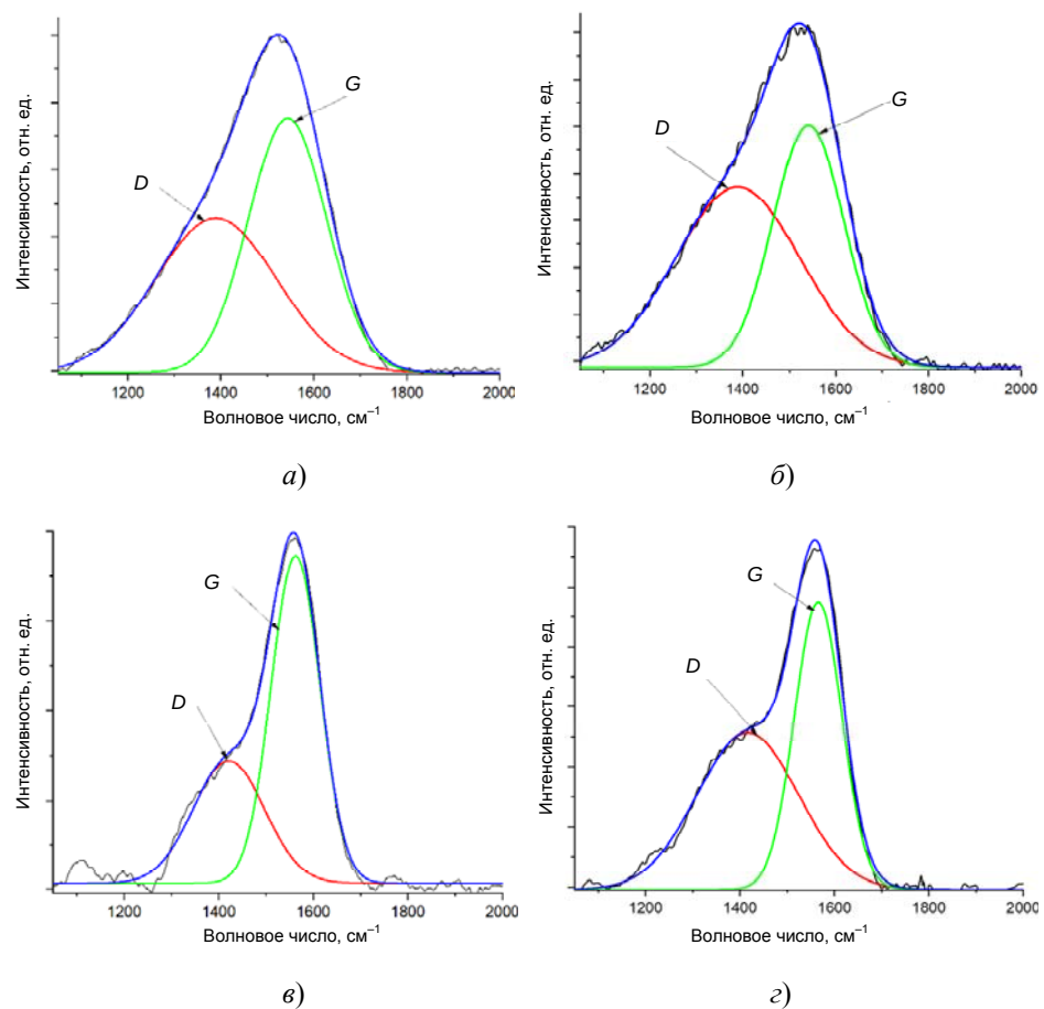
Рис. 5. КР-спектры медь-углеродных покрытий, осажденных путем импульсного испарения композиционного графит-медного катода и магнетронного испарения: а – КР-спектр в диапазоне от 1000 до 2000 \text{см}^{-1} для а-С : Си покрытия, осажденного при частоте 5 Гц; б – КР-спектр в диапазоне от 1000 до 2000 \text{см}^{-1} для а-С : Си покрытия, осажденного при частоте 15 Гц; в – КР-спектр в диапазоне от 1000 до 2000 \text{см}^{-1} для а-С : Си покрытия, полученного магнетронным испарением при частоте 5 кГц; г – КР-спектр в диапазоне от 1000 до 2000 \text{см}^{-1} для а-С : Си покрытия, осажденного магнетронным испарением при частоте 15 кГц
