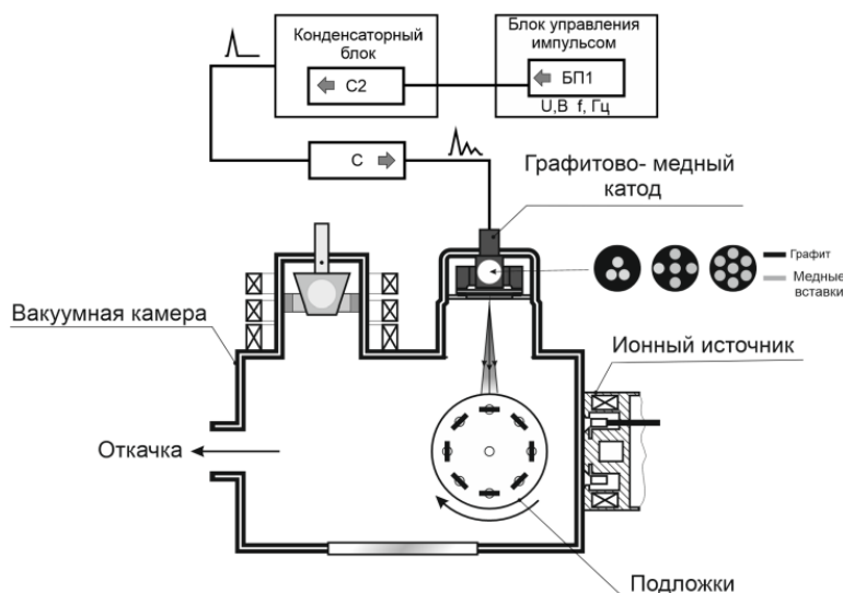
Рис. 2. Схема осаждения покрытий, за счет испарения составного медь-углеродного катода
