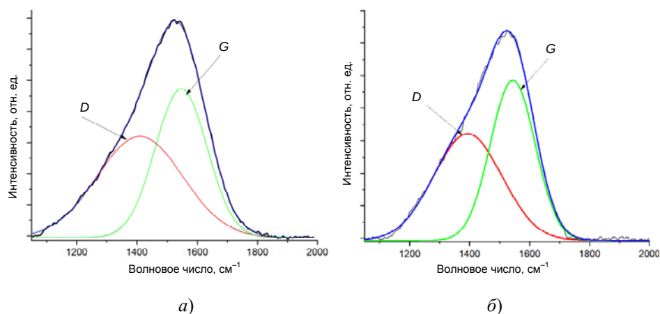
Рис. 4. КР-спектры медь-углеродных покрытий, осажденных из совмещенных потоков импульсной углеродной плазмы и потока меди, генерируемой дуговым разрядом постоянного тока: а – КР-спектр в диапазоне от 1000 до 2000 \text{см}^{-1} для а-С : Си покрытия, осажденного при частоте 5 Гц и токе дуги 80 А; б – КР-спектр в диапазоне от 1000 до 2000 \text{см}^{-1} для а-С : Си покрытия, осажденного при частоте 5 Гц и токе дуги 80 А
