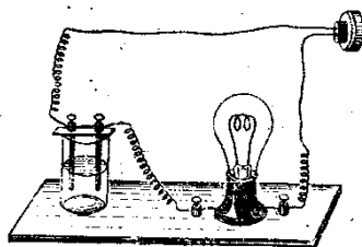
Рисунок 6.1 – Прибор для определения электропроводности раствора.
