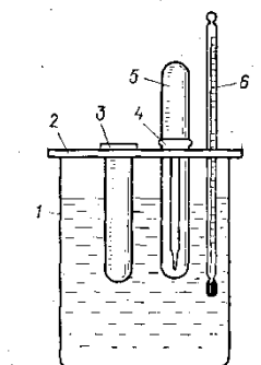
Рисунок 1.1 – Прибор для изучения зависимости скорости реакции от температуры:
