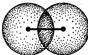
Рисунок 4.2– Схема перекрывания атомных 1s – электронных облаков при образовании молекулы H_2 .
