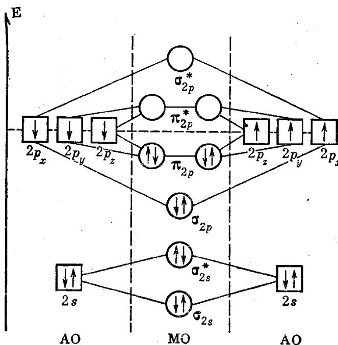
Рисунок 5.3 – Энергетическая схема образования молекулы азота.
