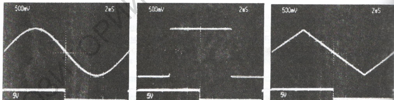
Рисунок 2 – Гармонический сигнал на выходе генератора, сигнал прямоугольной формы и сигнал треугольной формы.
