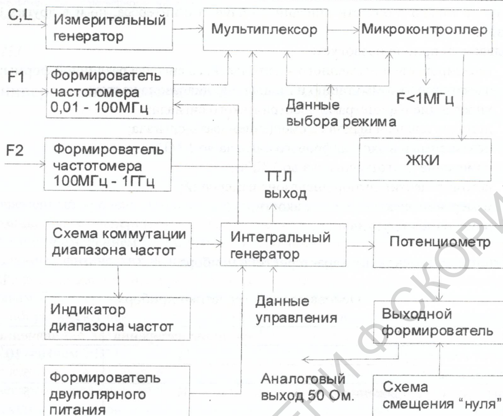
Рисунок 1 – Функциональная схема прибора
