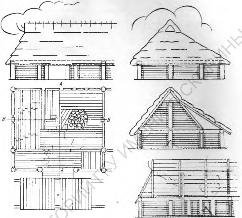
Рис. 11. Реконструкция плана сечения и внешнего вида домов
