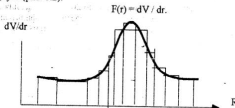
Рис 1.2. Дифференциальная кривая распределения пор по размерам
