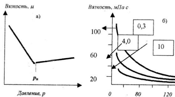
Рис. 3.1. Зависимость вязкости пластовой нефти от а) давления, б) растворенного газа и температуры (Цифры обозначают давление насыщения)
