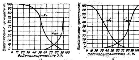
Рис.1.4. Зависимость относительных проницаемостей для жидкости и газа от водонасыщенности. а – песчаник; б – известняк и доломиты
