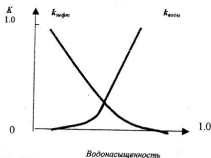
Рис.1.3. Относительная проницаемость песка для нефти и воды
