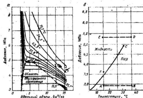
Рис. IV.1. Диаграмма фазового состояния чистого вещества
