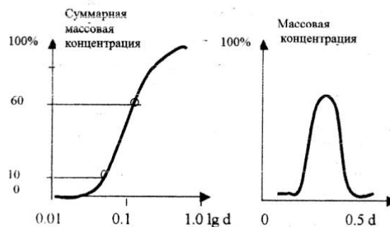
Рис. 1.1 Кривая гранулометрического состава породы.
