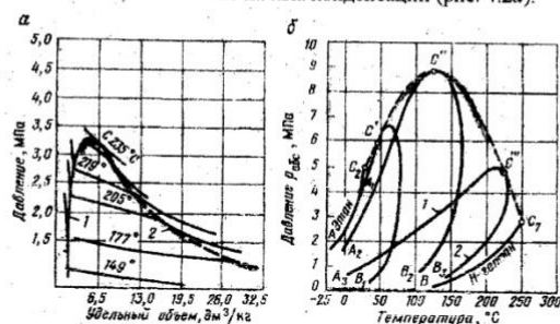
Рис. IV.2. Диаграммы фазового состояния двухкомпонентных систем. а — зависимость давления — удельный объем для смеси n -пентана и n -гептана, содержащей 52,4 % n -гептана; б — диаграммы давления — температура для смесей этана с n -гептаном (точки C' , C'' и C''' — критические точки смесей, содержащих соответственно 90,22, 50,35 и 9,6 % этана); 1 — линия точек начала парообразования; 2 — линия точек росы
