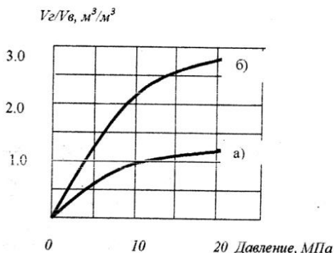
Рис. 3.7. Зависимость растворимости газов от давления
