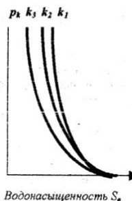
Рис. 1.6. Зависимость «капиллярное давление - водонасыщенность» пористых сред.
