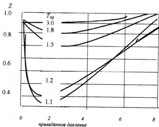
Рис. 3.5. Зависимость коэффициента сжимаемости природного газа от приведенного давления и температуры
