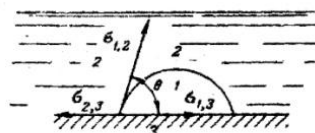
Рис. VI.4. Форма капли, обусловленная поверхностными натяжениями на различных границах соприкасающихся фаз.
