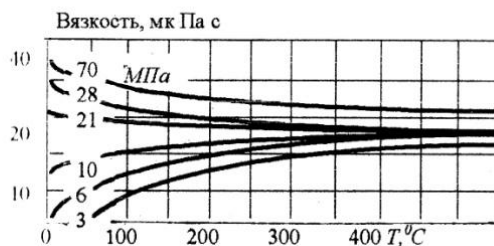
Рис.3.4. Зависимость коэффициента динамической вязкости метана от давления и температуры.
