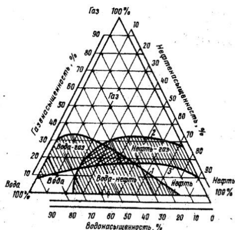
Рис. 1.5. Области распространения одно-, двух- и трехфазного потоков
