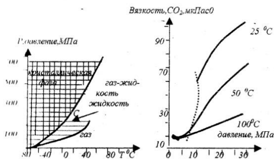
Рис. 5.4. Фазовая диаграмма углекислого газа
