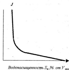
Рис. 1.7. Функция Леверетта для песчаника
