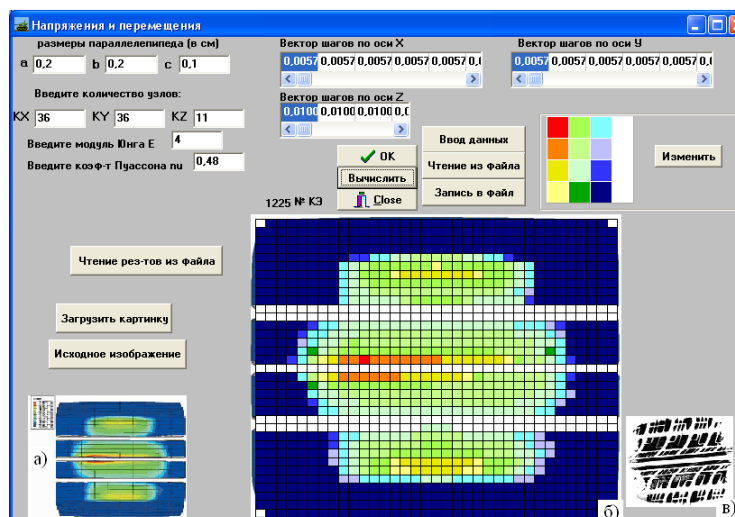
Рисунок 5. - Схема расчета при действии нагрузки (шины колеса) на основание: а)-численный расчет [8, 11].; б)- программная реализация; в)-эксперимент в черно-белом свете [9]
