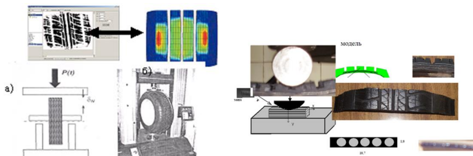
Рисунок 1. - Схемы и образцы испытаний, экспериментальные результаты, реализация численного исследования
