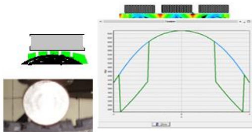
Рисунок 4. - Расчет напряжений при дискретном контакте. Графики зависимости \sigma_y от x при y = 3
