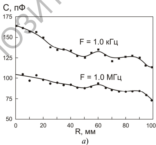
Рисунок 2.6 – Распределение емкости (а) и тангенса угла диэлектрических потерь (б) пленок оксида тантала
