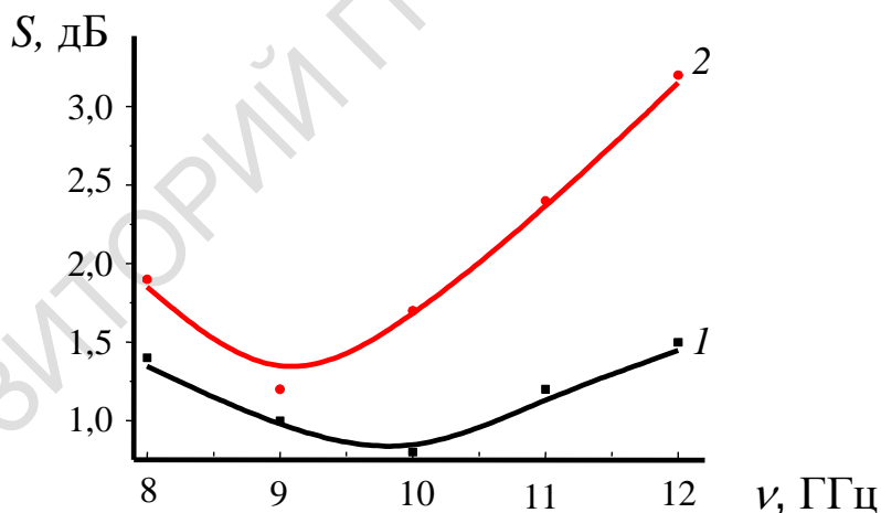
Рисунок 3 – Частотные зависимости ослабления S энергии ЭМИ, нормально падающего на образцы листовых пленочных СВЧ-поглоателей
