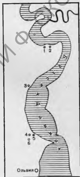
Рис. 1 Карта находок ольвийских монет на античных виллах побережья Бугского лимана: 1 — Дидова Хата, вилла № 1; 2 — Дидова Хата, вилла № 3; 3 — Козырка VIII, вилла № 1; 4 — Чертоватое II, вилла № 1; 5 — Чертоватое II, вилла № 3; 6 — Чертоватое II, вилла № 5
