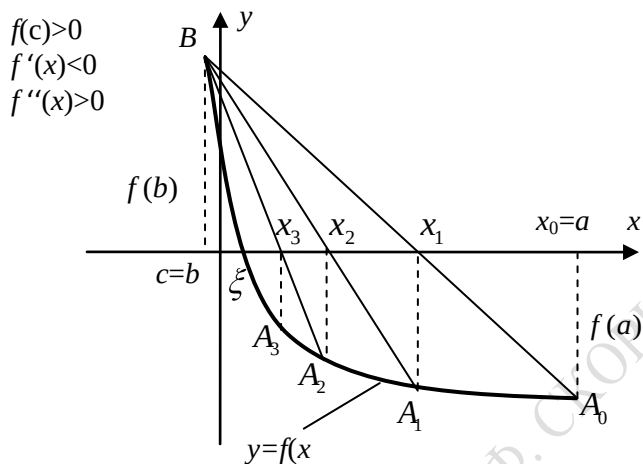
Рисунок 1.8 Иллюстрация метода хорд f(c) > 0 , f'(c) < 0
