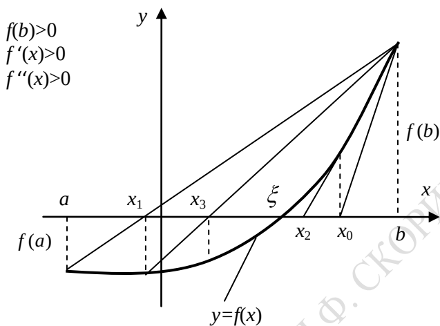
Рисунок 1.14 – Комбинированный метод f(b) > 0 , f'(x) > 0
