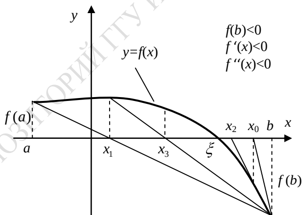
Рисунок 1.15 – Комбинированный метод f(b) < 0 , f'(x) < 0
