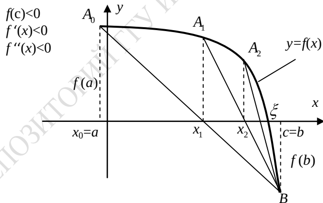
Рисунок 1.9 – Иллюстрация метода хорд f(c) < 0 , f'(c) < 0
