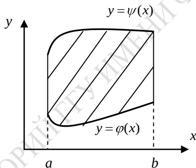
Рисунок 2.1 – Область интегрирования
