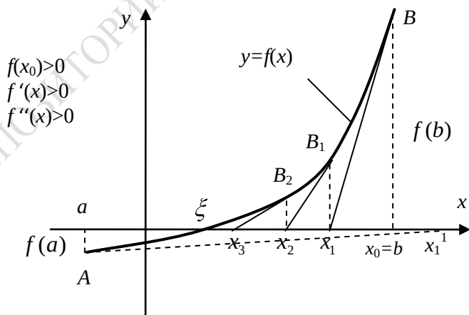
Рисунок 1.11 – Иллюстрация метода Ньютона
