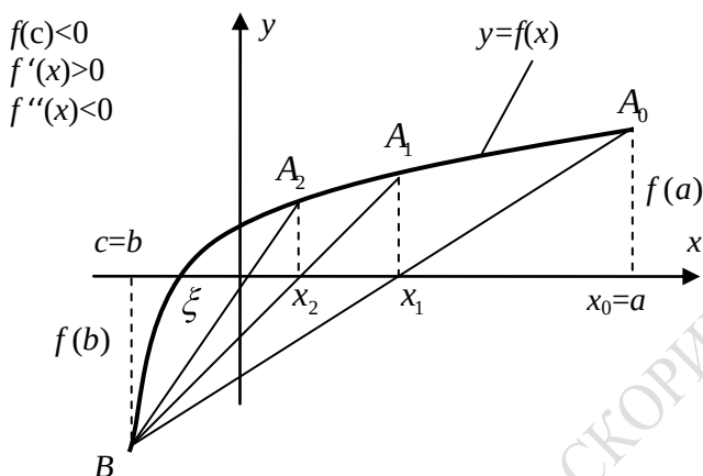
Рисунок 1.10 – Иллюстрация метода хорд f(c) < 0 , f'(c) > 0
