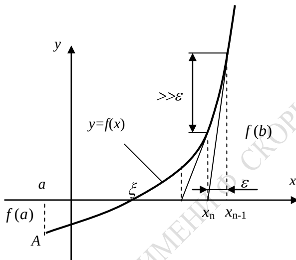
Рисунок 1.12 – О двух последовательных приближениях
