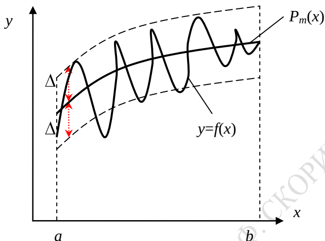
Рисунок 4.1 – Приближение функции
