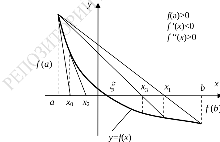
Рисунок 1.13 – Комбинированный метод f(a) > 0 , f'(x) < 0
