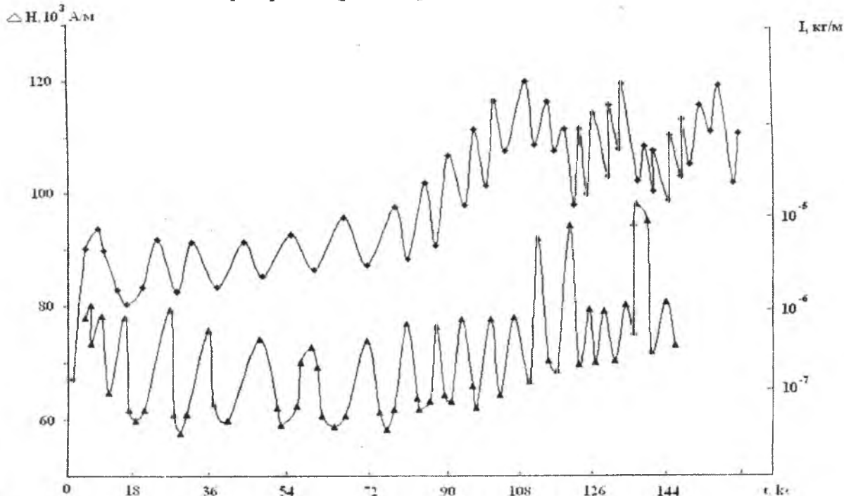
Рисунок 1– Зависимость ширины линии \Delta H ферромагнитного резонанса (1) и интенсивности изнашивания I (2) от времени трения t .
