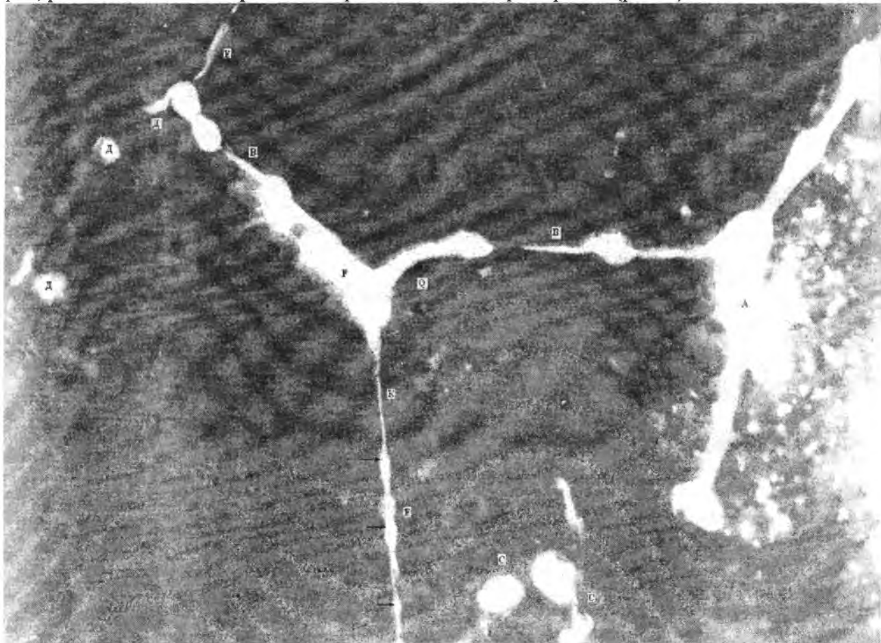
Рисунок 4 – Интеркристаллитное разрушение никеля. Время испытания 123,4 кс. Увеличение \times 54000 .
