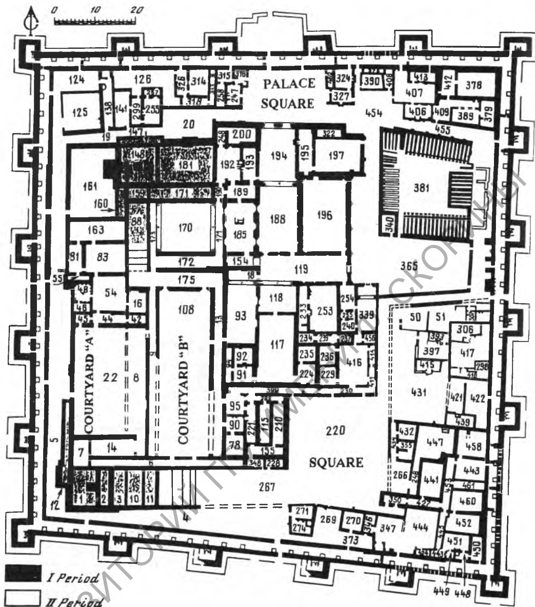
Рис. 2. Общий план дворца
