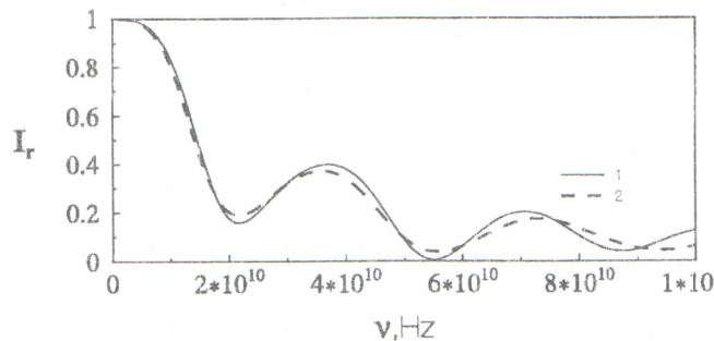
Рис. 1. График частотной зависимости интенсивности отраженной волны, если падающая волна поляризована вдоль оси X. 1 — для немагнитного диэлектрика, 2 — с учетом анизотропной магнитной проницаемости ( l = 5.5\text{мм} , \varepsilon_o = 4 + i0.8 , \varepsilon_e = 3 + i0.9 , \mu_1 = 1.0 , \mu_o = 1.1 , \mu_e = 1.3 , \lambda = 5.14 \cdot 10^{17} ).
