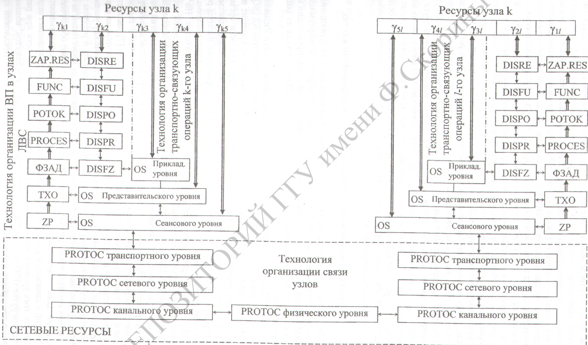
Рис. 1. Блок-схема технологии организации распределенной обработки информации и использования ресурсов сети ЭВМ
