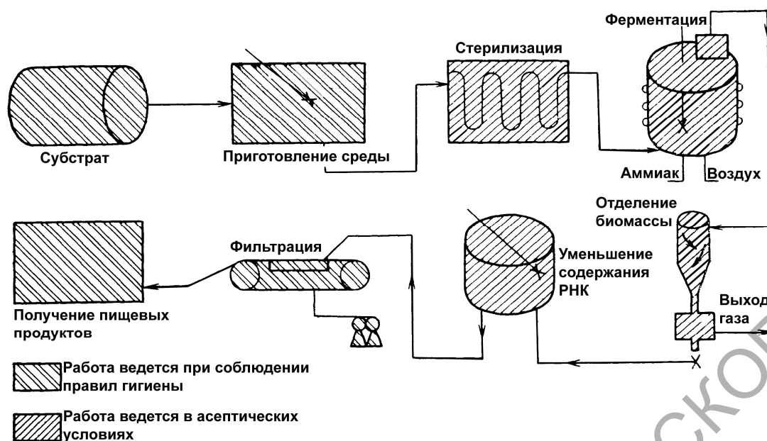
Рис. 4. Схематическое изображение производства микопротеина
