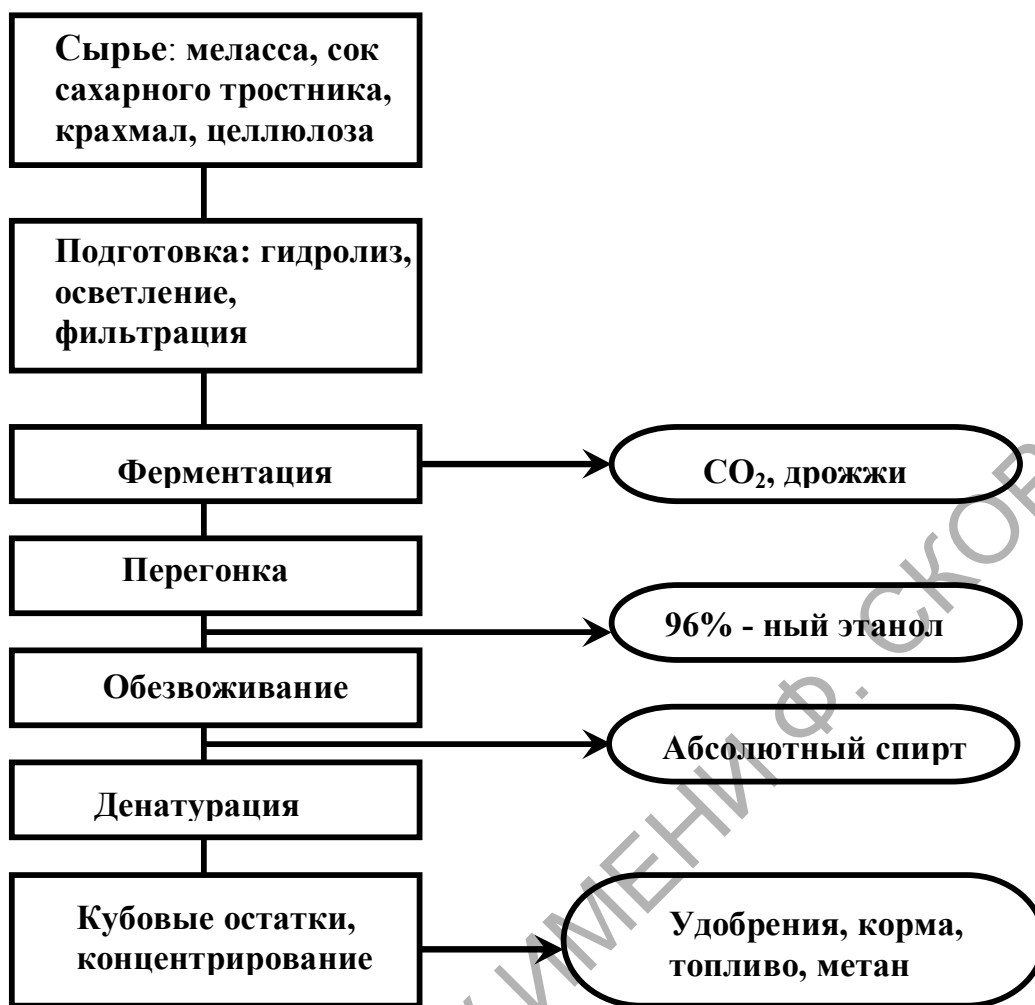
Рис. 6. Схема производства этанола
