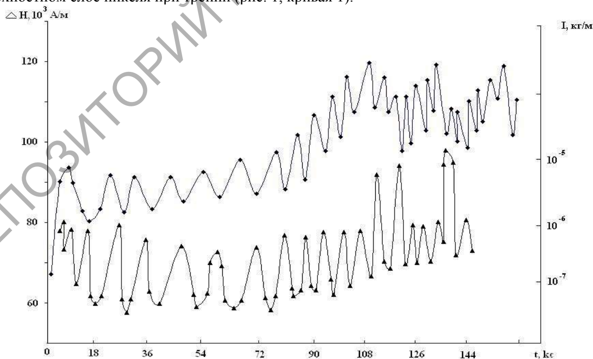
Рисунок 1– Зависимость ширины линии \Delta H ферромагнитного резонанса (1) и интенсивности изнашивания I (2) от времени трения t .
