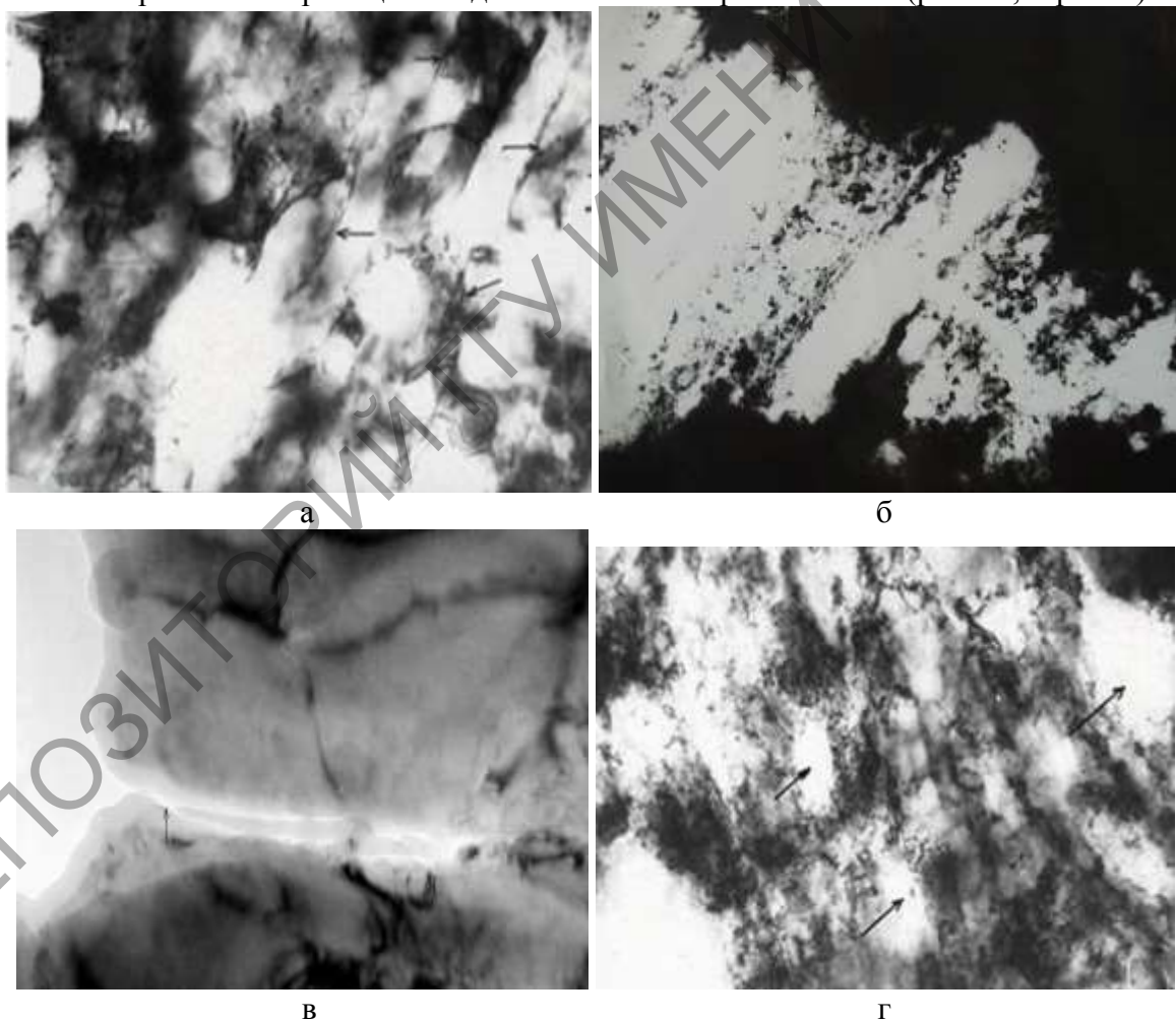
Рисунок 3 – Микроструктура транскристаллитного разрушения: а) – полосы структурного расслоения никеля ( t = 113,4 кс, стрелки); б) – трещины вдоль и поперёк полос скольжения ( t = 115,2 кс); в) – объединение микротрещин; г) – разрыхление материала за счёт пор ( t = 123 кс, стрелки).
