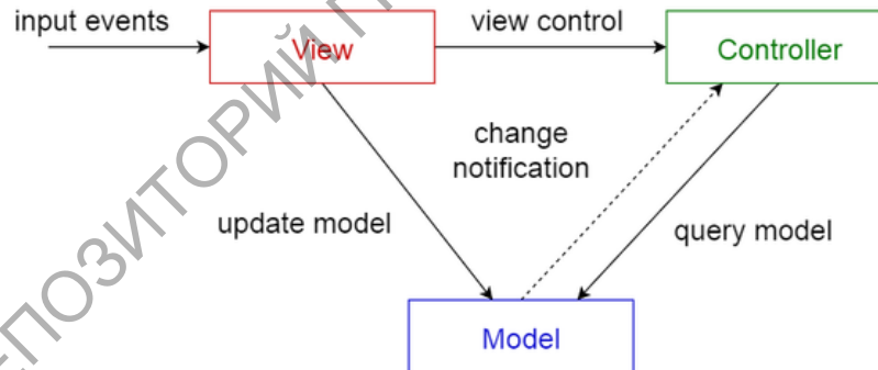
Рисунок 1 – Шаблон «Модель-Представление-Контроллер»
