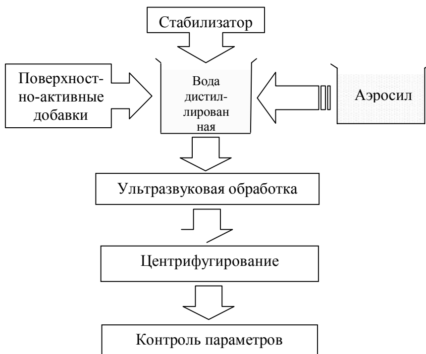
Рис. 1. Общая схема получения полирующих суспензий на основе диоксида кремния.
