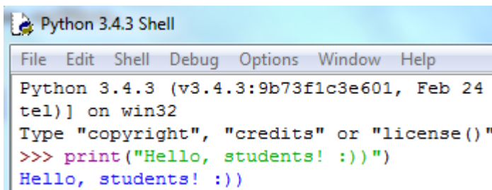
Рис. 1.3. Ввод-вывод сообщения
