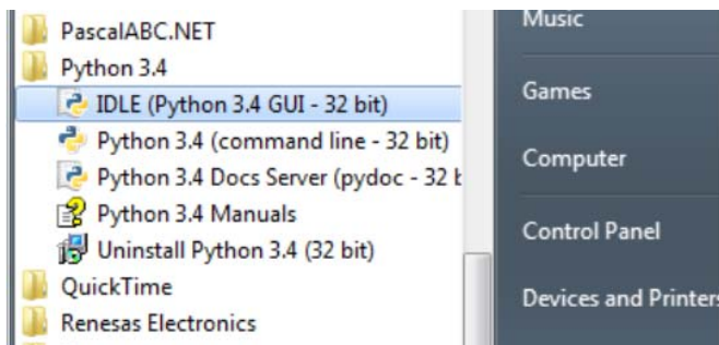
Рис. 1.2. Запуск IDLE
