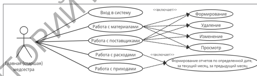
Рисунок 1 – Диаграмма вариантов использования приложения для главной медсестры
