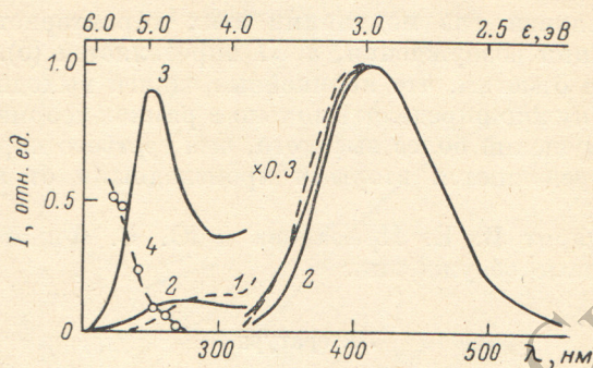
Рис. 1. Нормированные спектры РЛ (1—3) и возбуждения (4) кристалла LiF-TiO 2 при разных температурах. 1, 4 — 290, 2 — 80, 140, 3 — 63 К.
